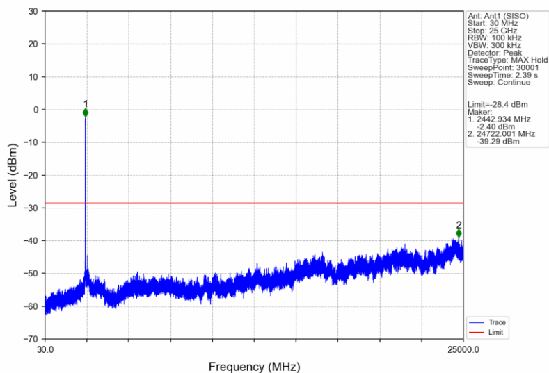
802.11g_MCH_2437MHz_Ant1 (SISO)_NTNV
