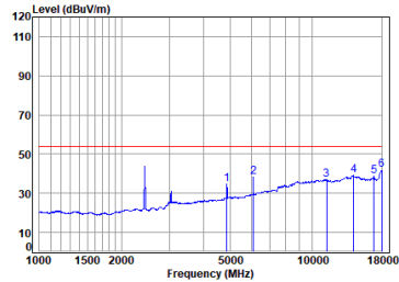
11g_TX_CH_06_Vertical-Avg
