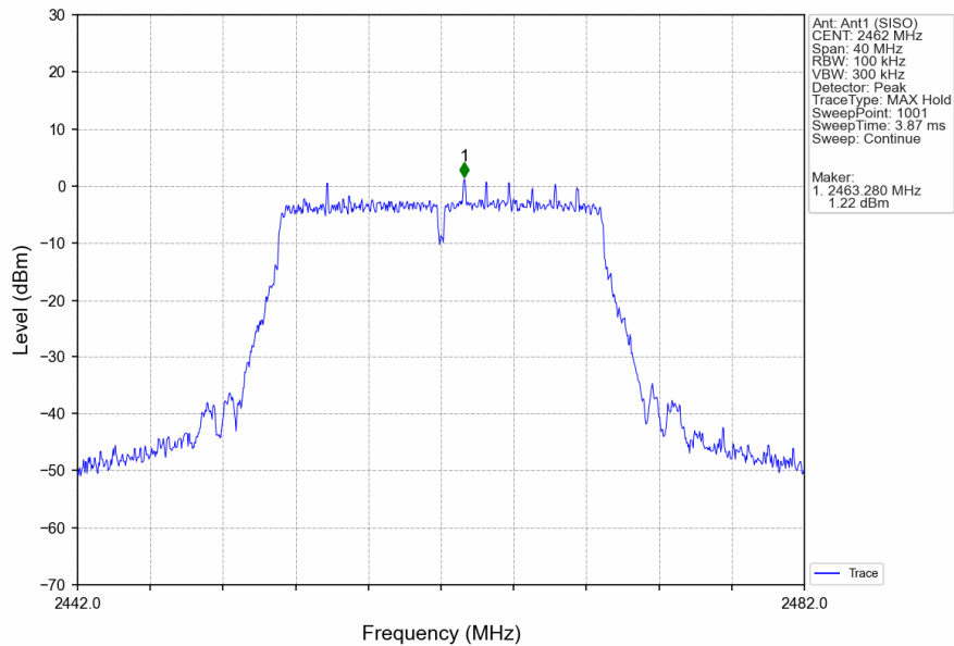
802.11n(HT20)_HCH_2462MHz_Ant1 (SISO)_NTNW
