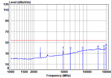
11g_TX_CH_06_Horizontal-Avg
