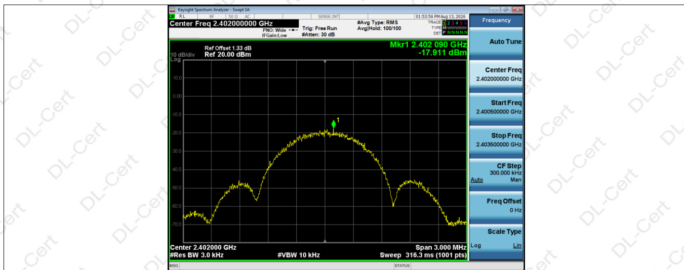
PSD NVNT BLE 1M 2402MHz Ant1
