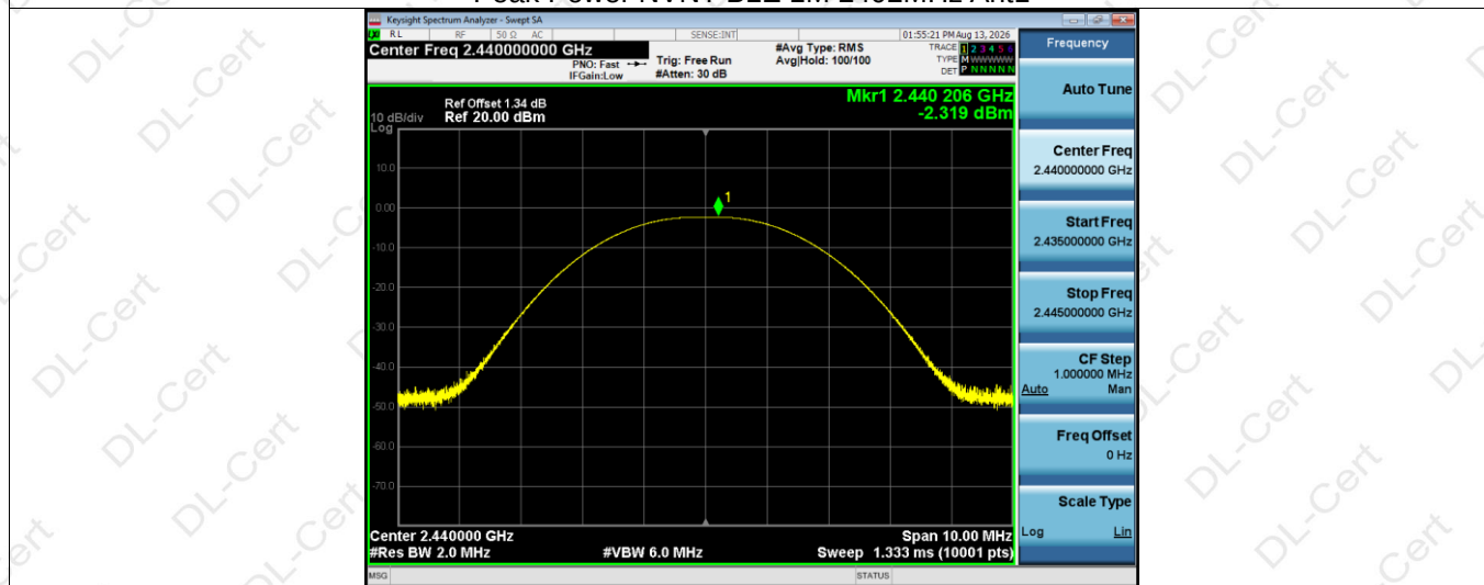
Peak Power NVNT BLE 1M 2440MHz Ant1
