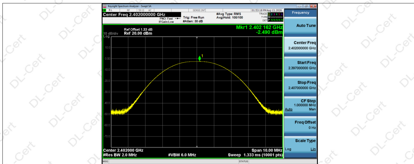
Peak Power NVNT BLE 1M 2402MHz Ant1
