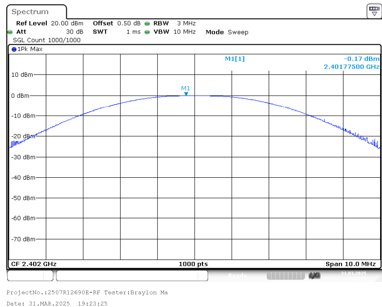
BLE 1Mbps Low Channel
