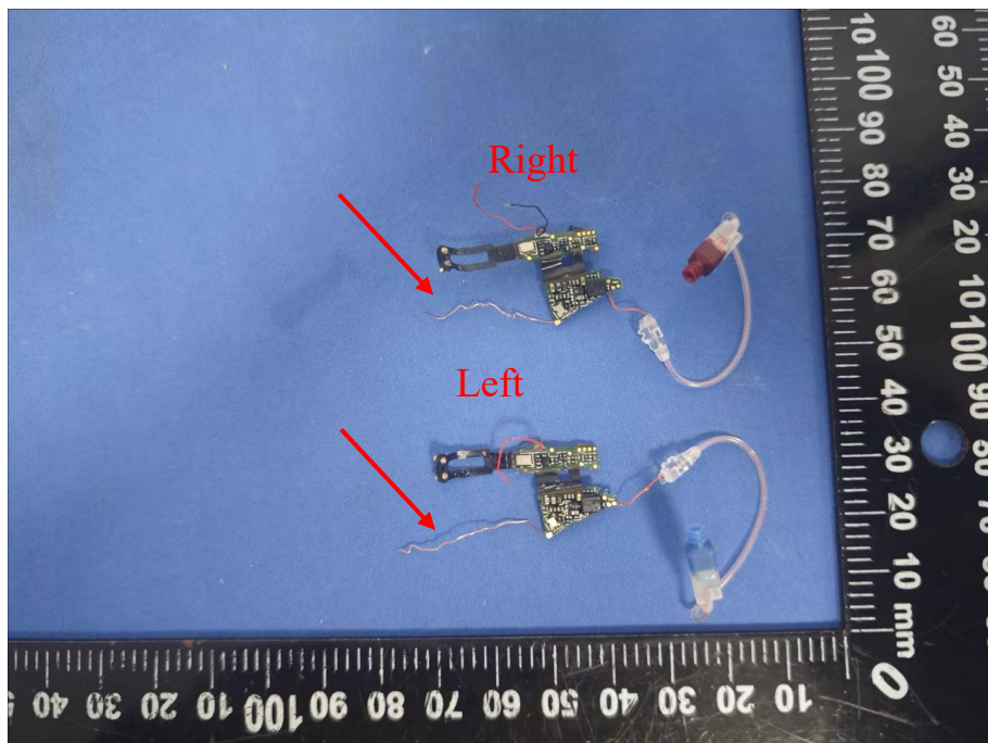
BLE/BT Antenna
