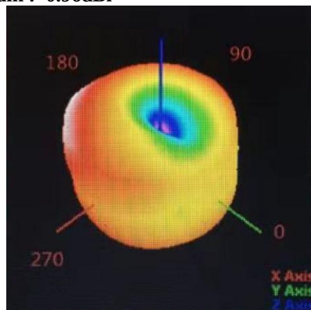
2480MHz \phi=0^\circ , \theta=0^\circ
