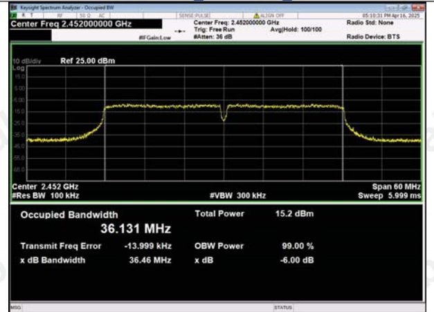
IEEE 802.11n_Channel 9_40MHz
