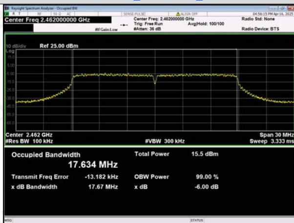
IEEE 802.11n_Channel 11_20MHz
