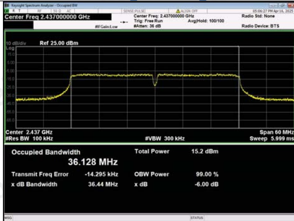
IEEE 802.11n_Channel 6_40MHz
