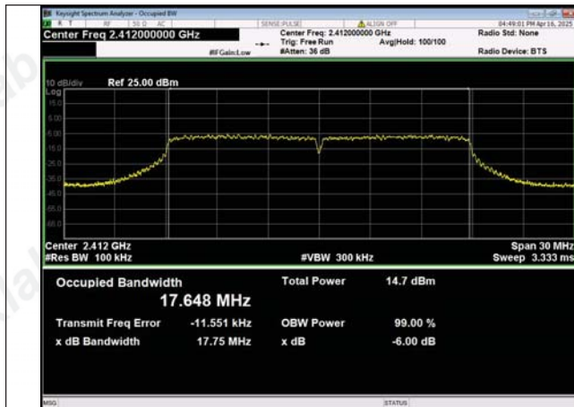
IEEE 802.11n_Channel 1_20MHz
