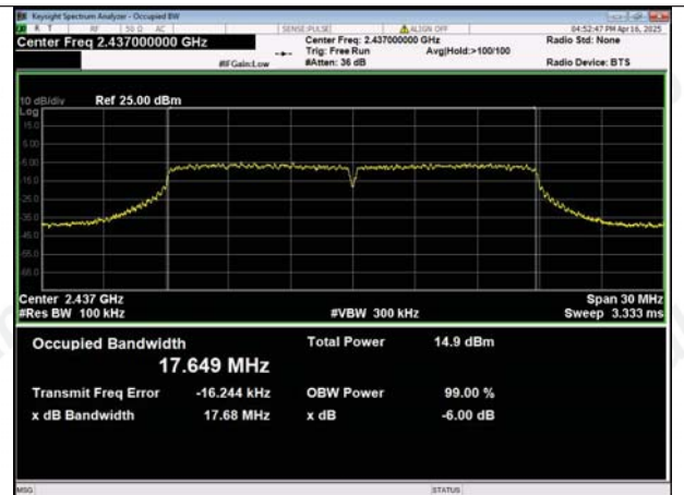
IEEE 802.11n_Channel 6_20MHz
