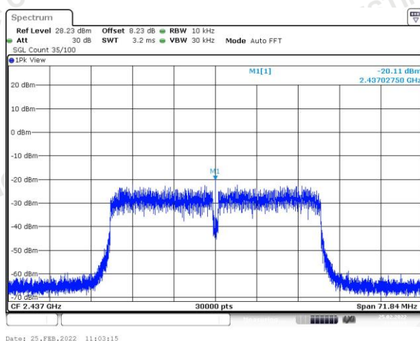
CH06
