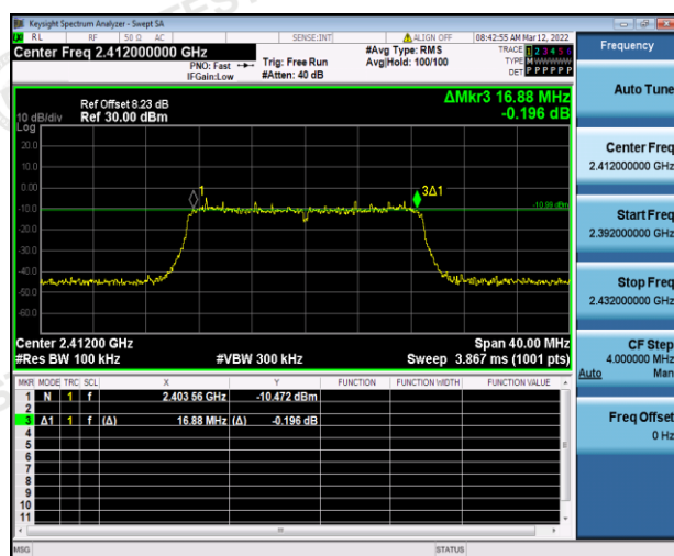
CH01
