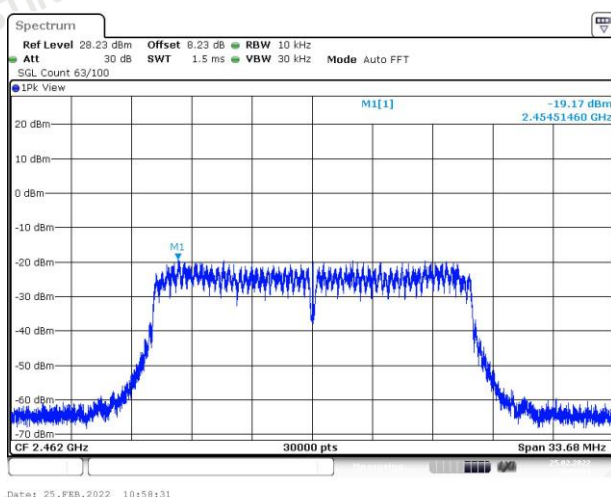
CH11
