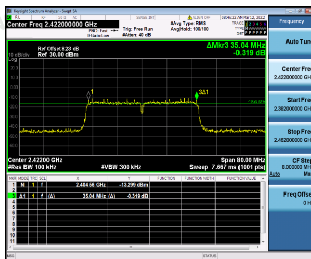
CH03
