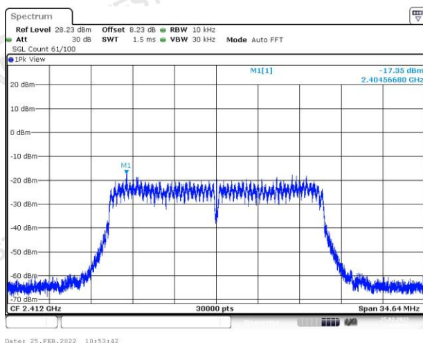
CH01
