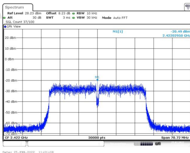
CH03
