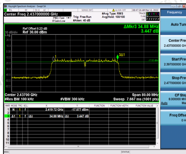
CH06
