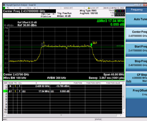
CH06
