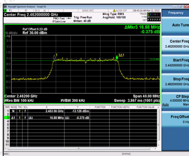
CH11
