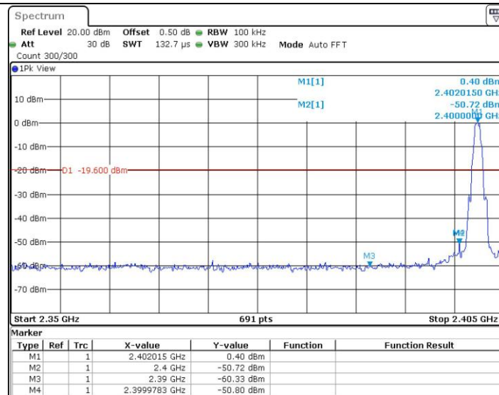
BLE_Low_2402
