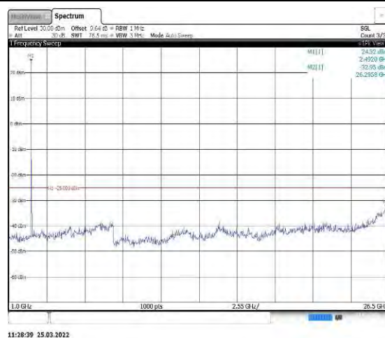
Band7-20MHz-QPSK-20850-1RB#0-Range2: 1000~26500MHz
