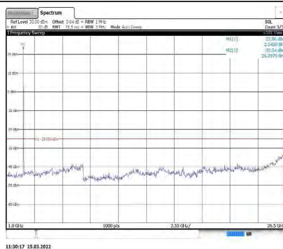
Band7-20MHz-QPSK-21350-1RB#0-Range2: 1000~26500MHz
