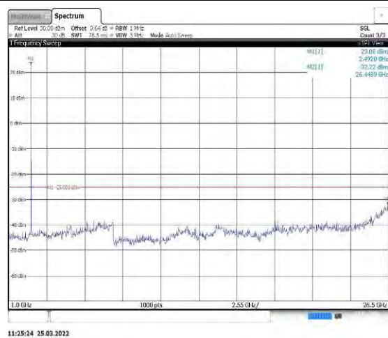
Band7-15MHz-QPSK-20825-1RB#0-Range2: 1000~26500MHz
