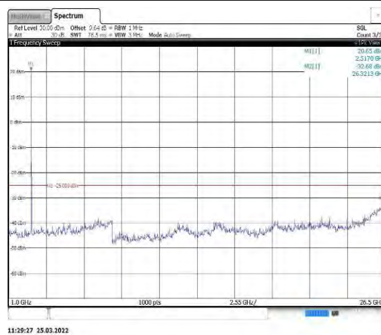
Band7-20MHz-QPSK-21100-1RB#0-Range2: 1000~26500MHz
