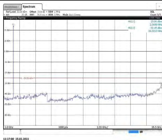
Band7-15MHz-QPSK-21100-1RB#0-Range2: 1000~26500MHz
