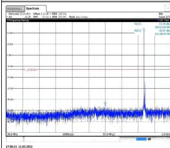
Band26-10MHz-16QAM-26990-1RB#0-Rang e1:30~1000MHz
