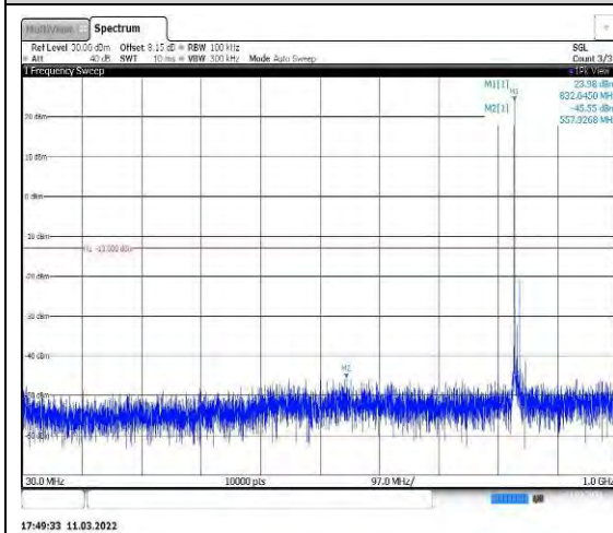
Band26-10MHz-16QAM-26915-1RB#0-Rang e1:30~1000MHz
