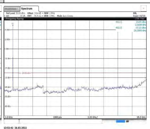
Band38-5MHz-QPSK-37775-1RB#0-Range2:1 000~26500MHz
