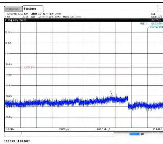
Band26-5MHz-QPSK-26715-1RB#0-Range2: 1000~10000MHz
