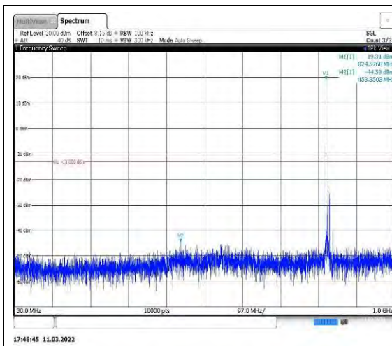
Band26-10MHz-16QAM-26840-1RB#0-Rang e1:30~1000MHz
