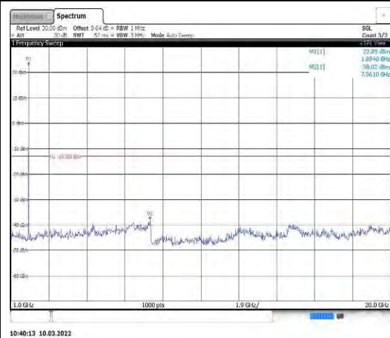
Band25-5MHz-QPSK-26365-1RB#0-Range2: 1000~20000MHz
