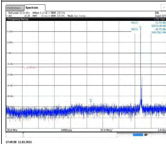
Band26-10MHz-QPSK-26990-1RB#0-Range 1:30~1000MHz
