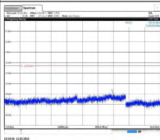
Band26-5MHz-QPSK-26765-1RB#0-Range2: 1000~10000MHz
