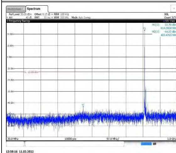
Band26-10MHz-16QAM-26740-1RB#0-Rang e1:30~1000MHz
