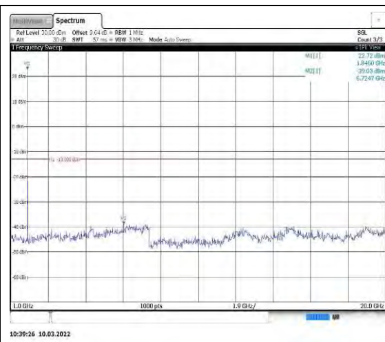
Band25-5MHz-QPSK-26065-1RB#0-Range2: 1000~20000MHz
