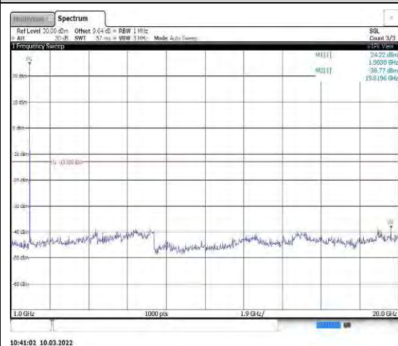
Band25-5MHz-QPSK-26665-1RB#0-Range2: 1000~20000MHz
