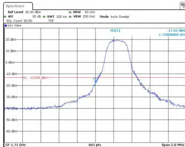
Band4-3MHz-QPSK-19965-1RB#14
