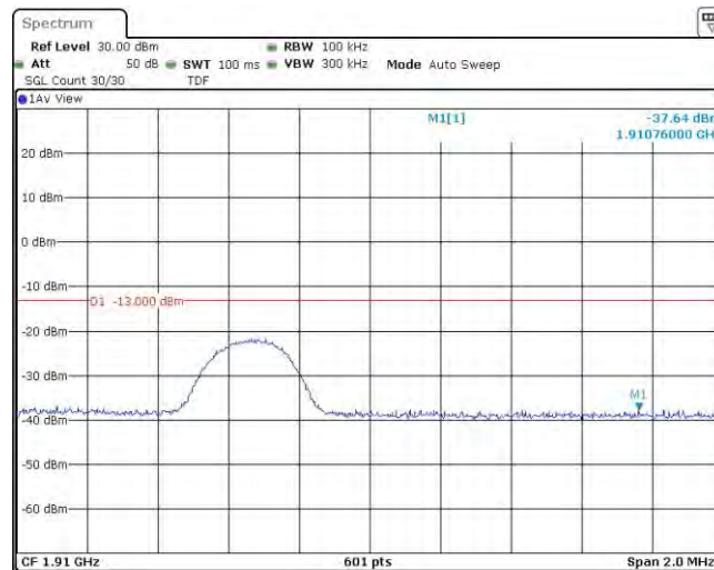
Band2-5MHz-QPSK-19175-1RB#24
