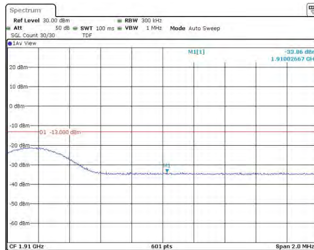
Band2-15MHz-16QAM-19125-1RB#74
