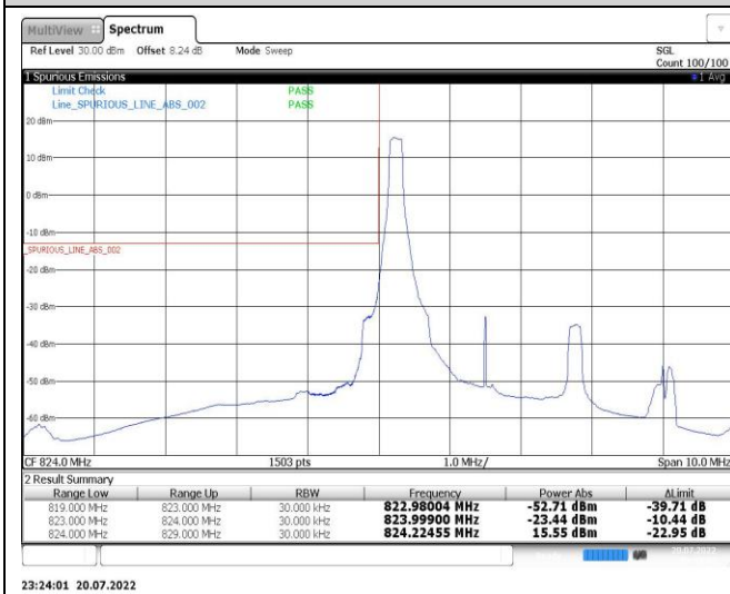
Band5-3MHz-QPSK-20635-1RB#14
