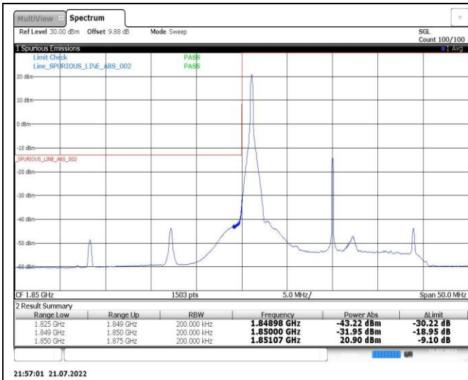
Band25-20MHz-16QAM-26590-1RB#99
