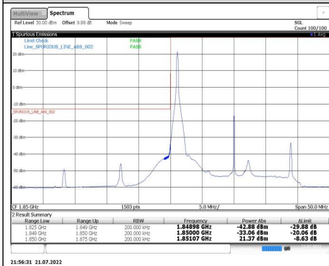
Band25-20MHz-QPSK-26590-1RB#99
