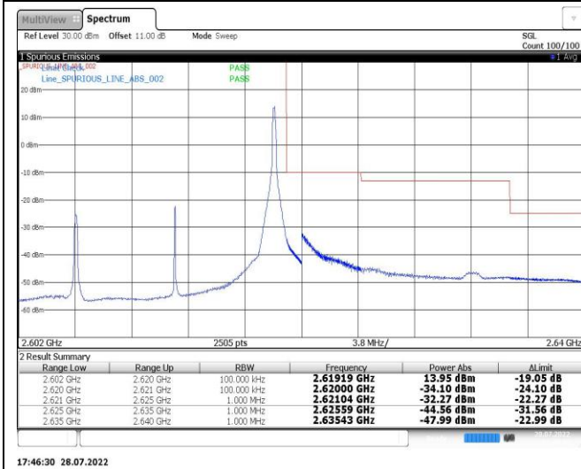
Band38-20MHz-QPSK-37850-1RB#0
