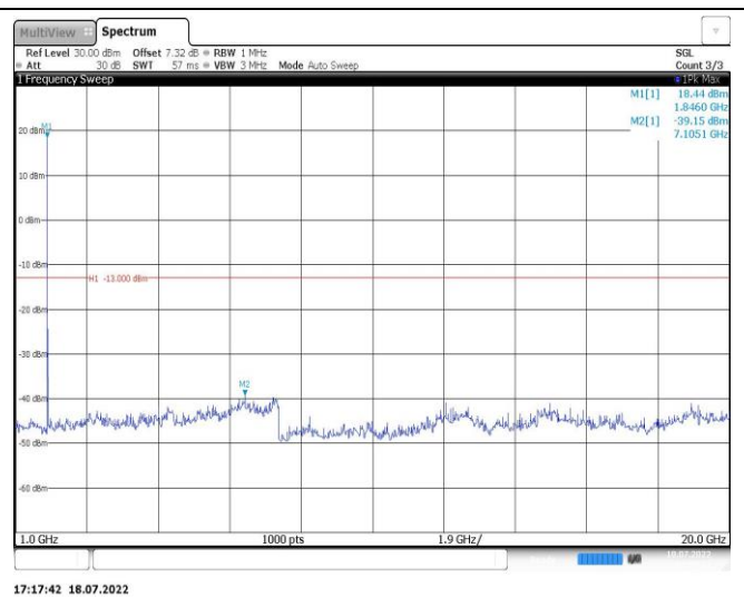
Band2-5MHz-QPSK-18900-1RB#0-Range2:1000~20000MHz
