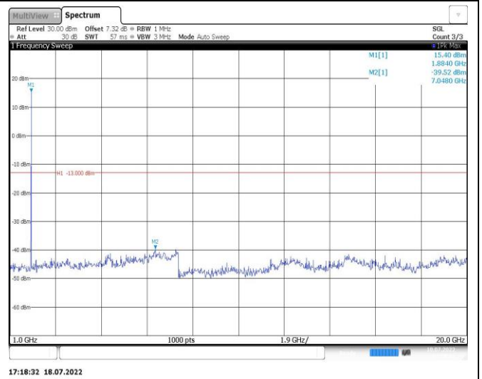
Band2-5MHz-16QAM-19175-1RB#0-Range2:1000~20000MHz
