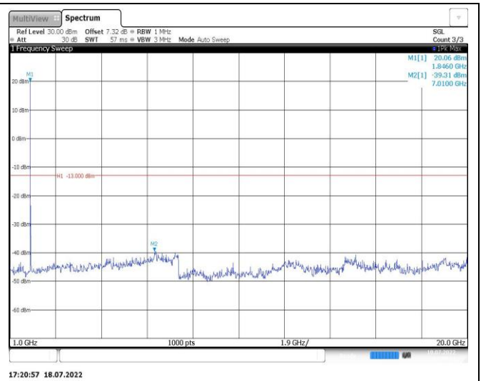
Band2-10MHz-QPSK-18900-1RB#0-Range2:1000~20000MHz
