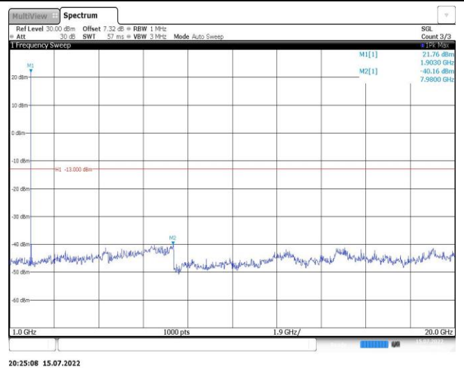
Band2-3MHz-QPSK-18615-1RB#0-Range2:1000~20000MHz
