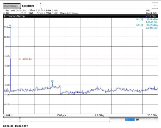
Band2-3MHz-QPSK-19185-1RB#0-Range2:1000~20000MHz
