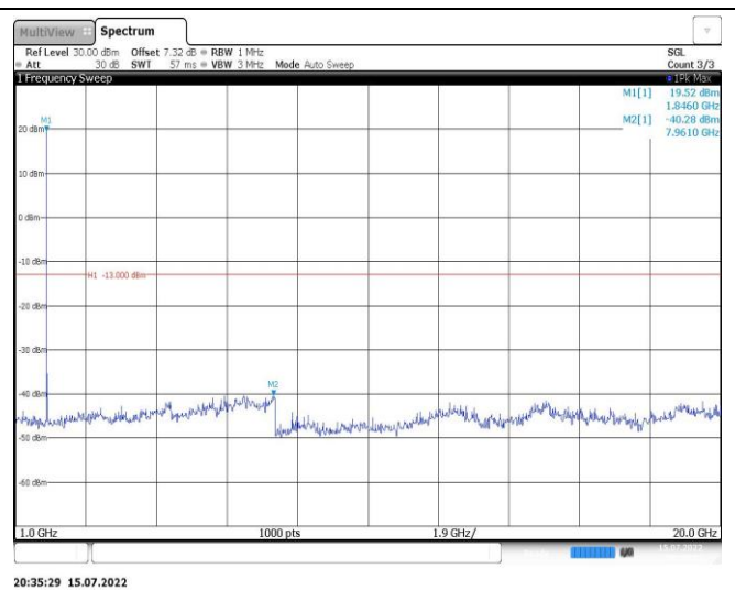
Band2-3MHz-QPSK-18900-1RB#0-Range2:1000~20000MHz
