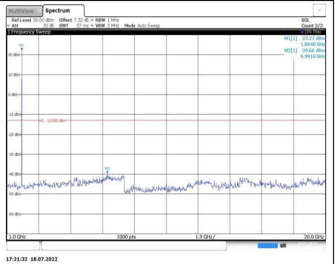
Band2-10MHz-QPSK-19150-1RB#0-Range2:1000~20000MHz
