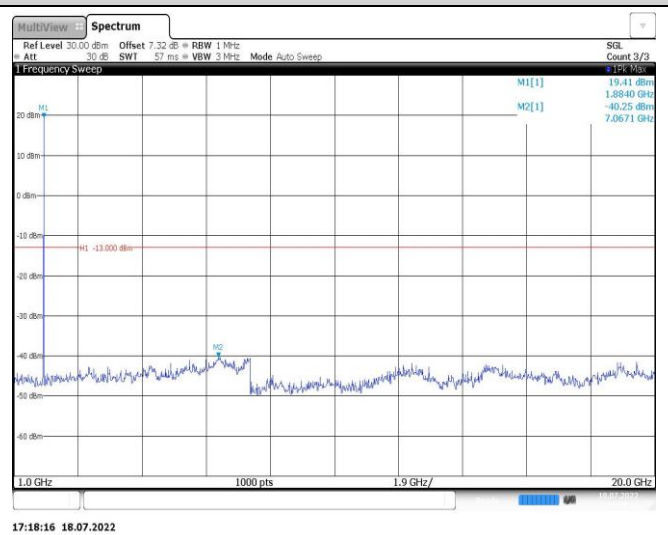
Band2-5MHz-QPSK-19175-1RB#0-Range2:1000~20000MHz
