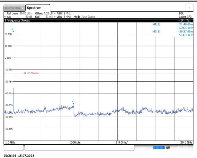
Band2-3MHz-16QAM-18615-1RB#0-Range2:1000~20000MHz
