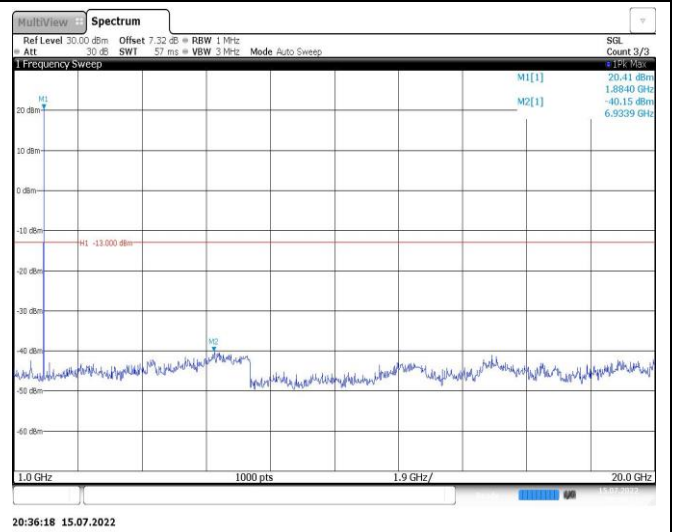
Band2-3MHz-16QAM-19185-1RB#0-Range2:1000~20000MHz
