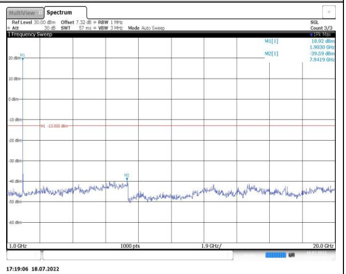
Band2-10MHz-QPSK-18650-1RB#0-Range2:1000~20000MHz
