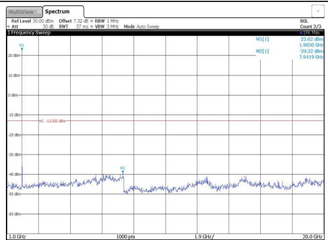
Band2-1.4MHz-QPSK-19193-1RB#0-Range2:1000~20000MHz
