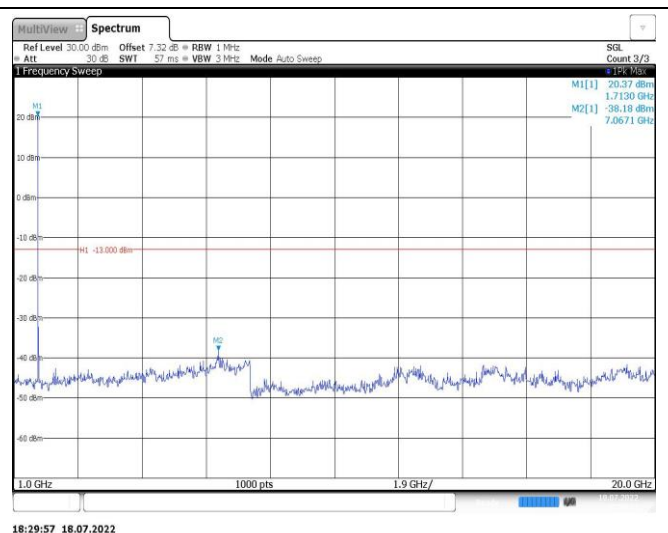
Band4-10MHz-QPSK-20175-1RB#0-Range2:1000~20000MHz
