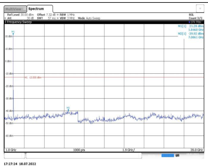
Band2-20MHz-QPSK-18900-1RB#0-Range2:1000~20000MHz
