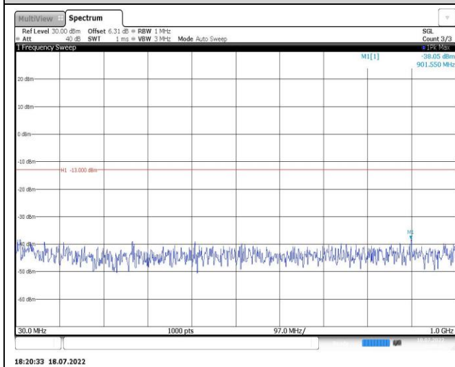
Band4-1.4MHz-QPSK-20393-1RB#0-Range1:30~1000MHz
