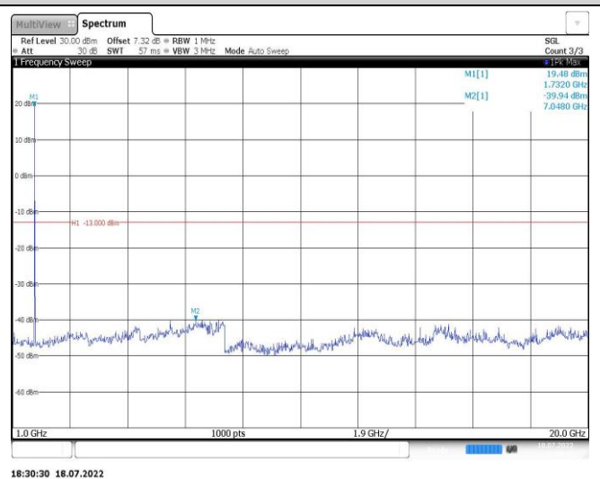
Band4-10MHz-QPSK-20350-1RB#0-Range2:1000~20000MHz
