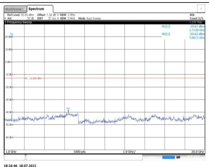
Band4-5MHz-QPSK-20175-1RB#0-Range2:1000~20000MHz
