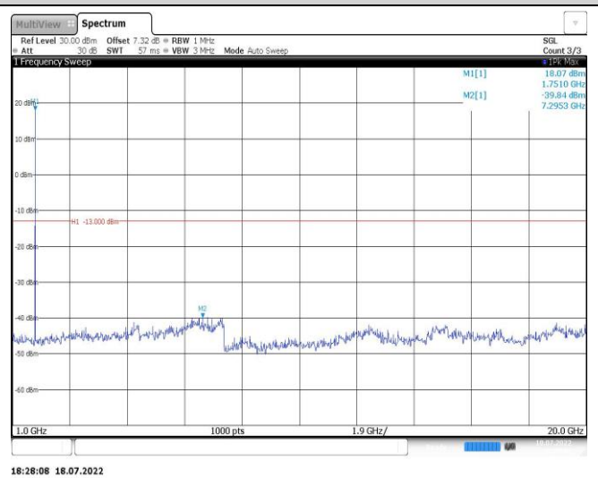
Band4-10MHz-QPSK-20000-1RB#0-Range2:1000~20000MHz
