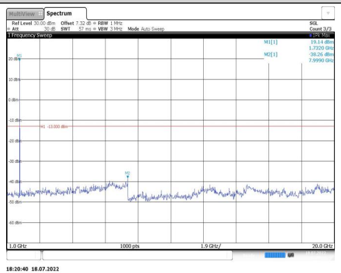
Band4-1.4MHz-QPSK-20393-1RB#0-Range2:1000~20000MHz
