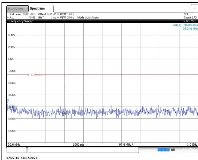
Band2-20MHz-QPSK-18900-1RB#0-Range1:30~1000MHz
