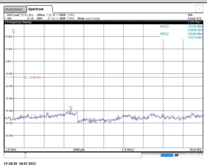
Band2-20MHz-16QAM-18700-1RB#0-Range2:1000~20000MHz
