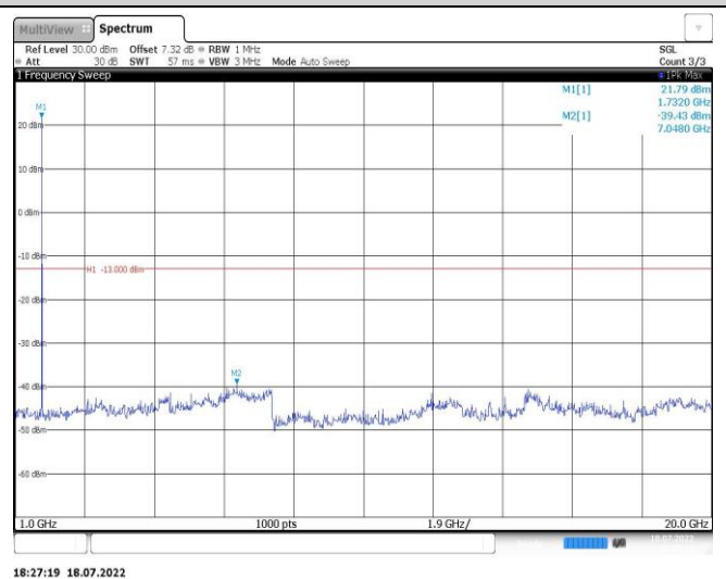
Band4-5MHz-QPSK-20375-1RB#0-Range2:1000~20000MHz
