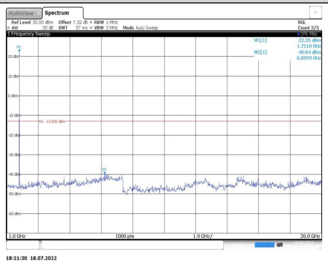
Band4-3MHz-QPSK-19965-1RB#0-Range2:1000~20000MHz
