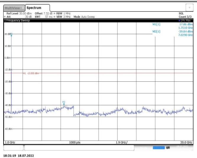
Band4-15MHz-QPSK-20025-1RB#0-Range2:1000~20000MHz
