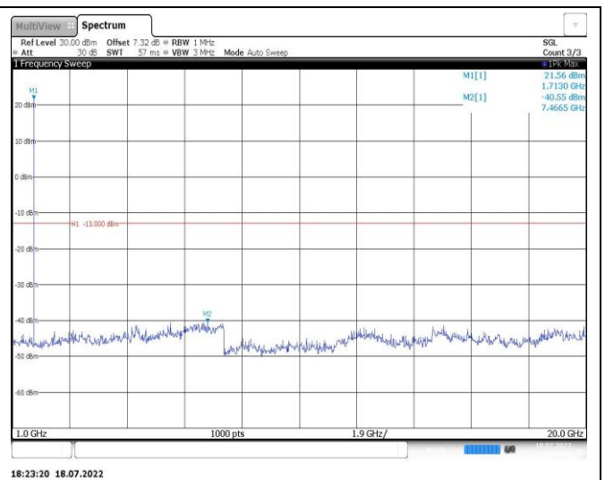
Band4-3MHz-QPSK-20175-1RB#0-Range2:1000~20000MHz
