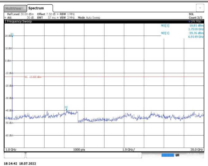
Band4-5MHz-QPSK-19975-1RB#0-Range2:1000~20000MHz
