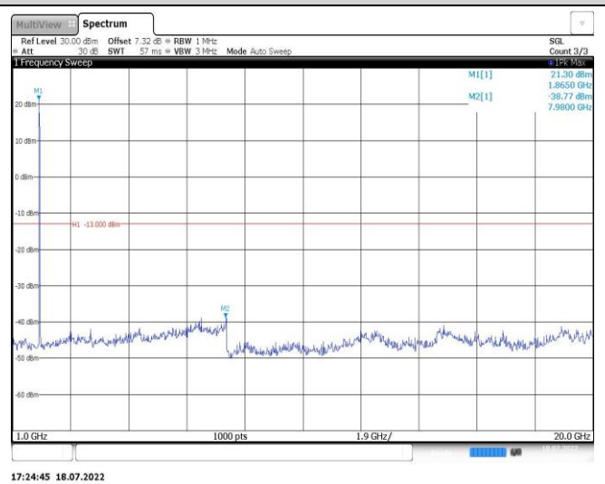
Band2-15MHz-QPSK-19125-1RB#0-Range2:1000~20000MHz
