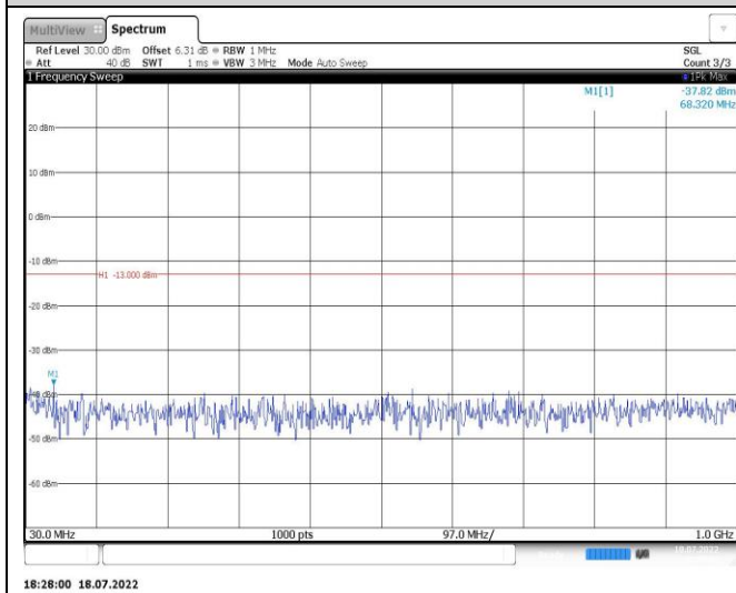
Band4-10MHz-QPSK-20000-1RB#0-Range1:30~1000MHz
