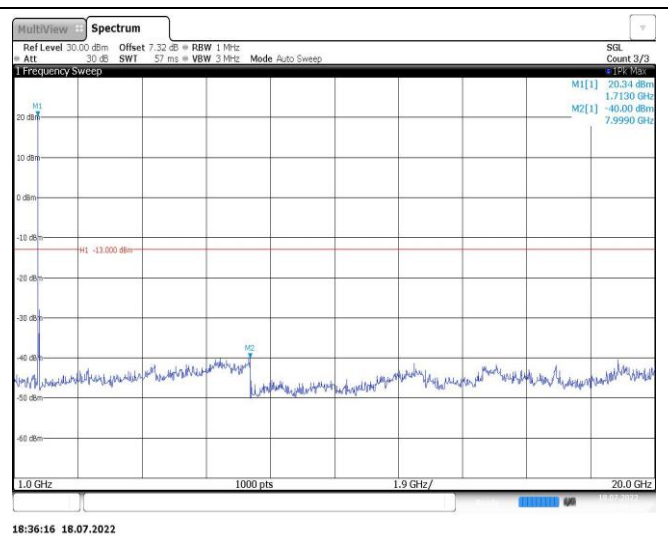
Band4-20MHz-QPSK-20175-1RB#0-Range2:1000~20000MHz
