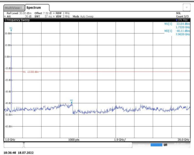
Band4-20MHz-QPSK-20300-1RB#0-Range2:1000~20000MHz
