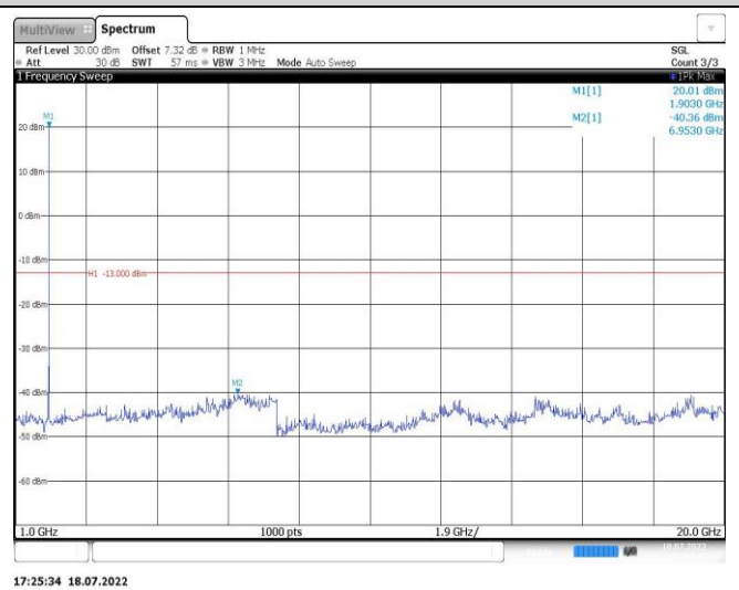
Band2-20MHz-QPSK-18700-1RB#0-Range2:1000~20000MHz
