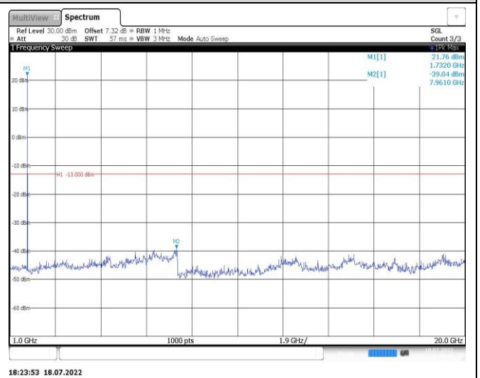
Band4-3MHz-QPSK-20385-1RB#0-Range2:1000~20000MHz
