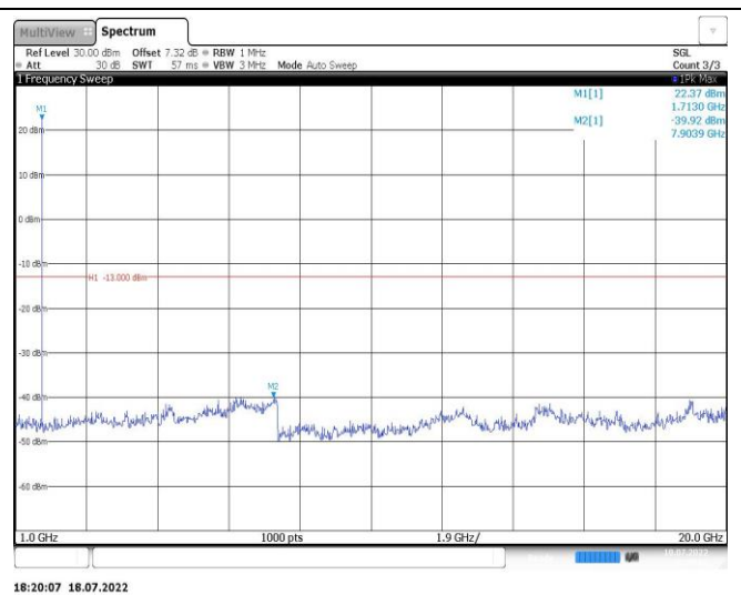
Band4-1.4MHz-QPSK-20175-1RB#0-Range2:1000~20000MHz
