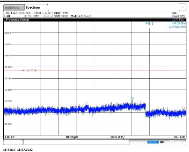
Band5-3MHz-QPSK-20415-1RB#0-Range2:1000~10000MHz
