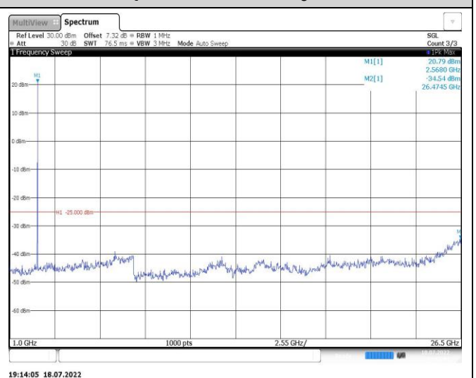
Band7-10MHz-16QAM-20800-1RB#0-Range2:1000~26500MHz
