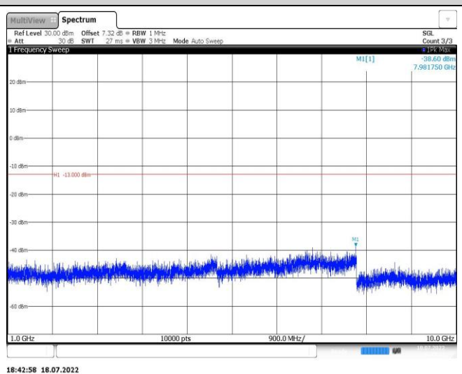
Band5-3MHz-QPSK-20635-1RB#0-Range2:1000~10000MHz
