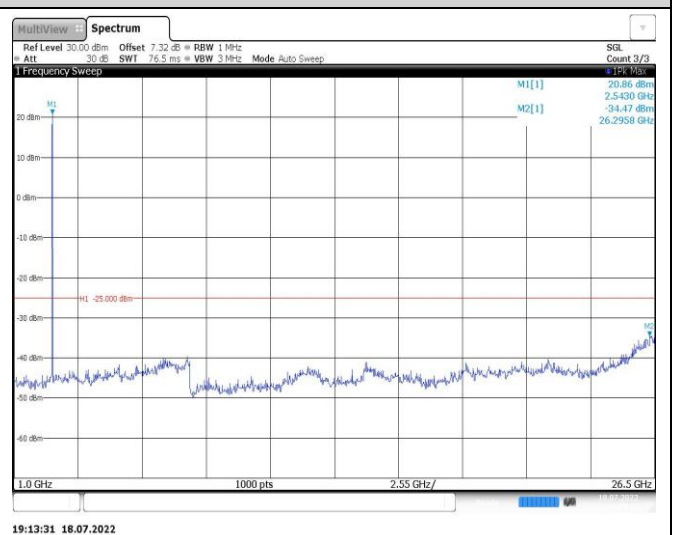
Band7-10MHz-QPSK-21400-1RB#0-Range2:1000~26500MHz
