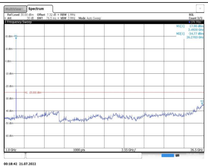
Band7-5MHz-QPSK-21100-1RB#0-Range2:1000~26500MHz
