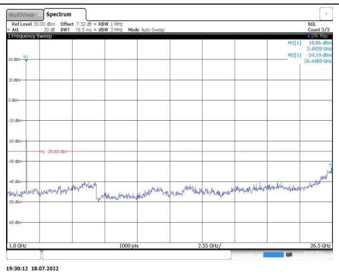
Band7-20MHz-QPSK-21100-1RB#0-Range2:1000~26500MHz
