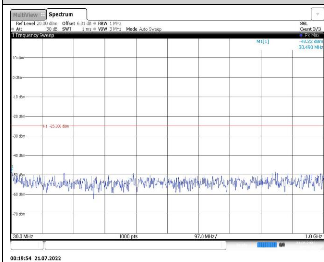
Band7-10MHz-QPSK-20800-1RB#0-Range1:30~1000MHz
