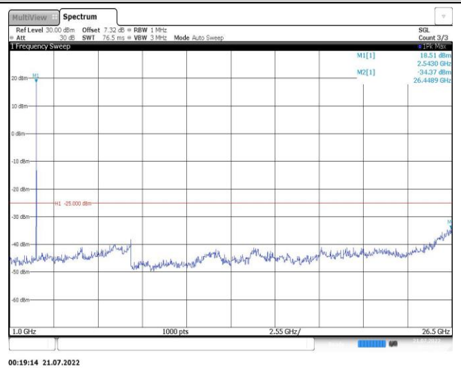
Band7-5MHz-QPSK-21425-1RB#0-Range2:1000~26500MHz
