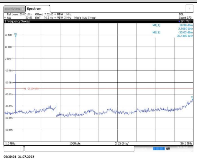
Band7-10MHz-QPSK-20800-1RB#0-Range2:1000~26500MHz
