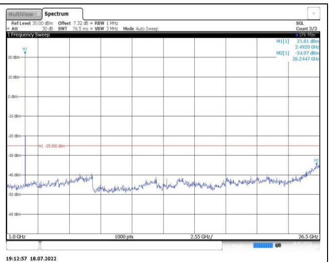
Band7-10MHz-QPSK-21100-1RB#0-Range2:1000~26500MHz
