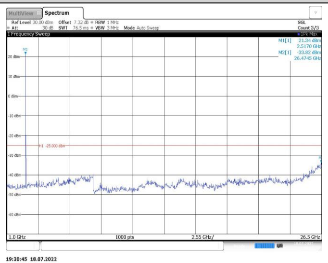
Band7-20MHz-QPSK-21350-1RB#0-Range2:1000~26500MHz
