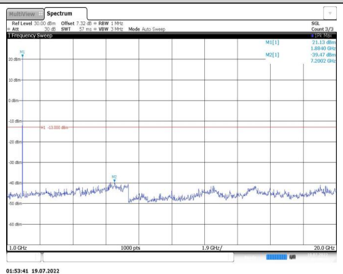
Band25-3MHz-QPSK-26675-1RB#0-Range2:1000~20000MHz
