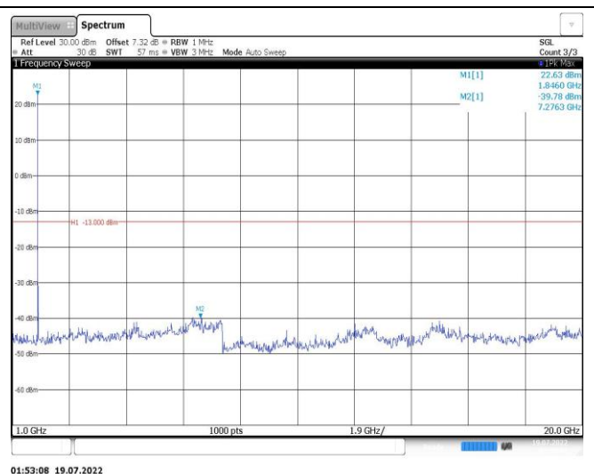
Band25-3MHz-QPSK-26365-1RB#0-Range2:1000~20000MHz
