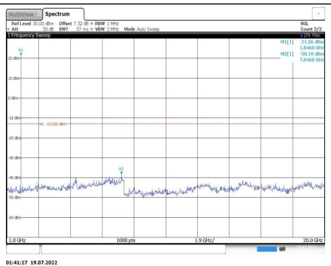
Band25-1.4MHz-QPSK-26365-1RB#0-Range2:1000~20000MHz
