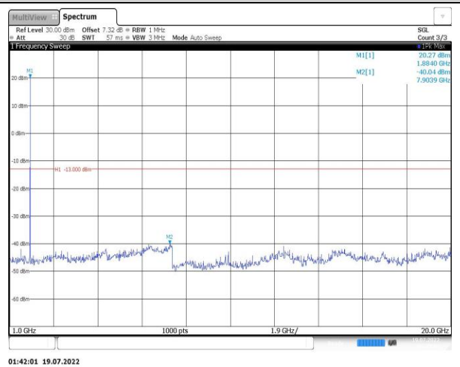
Band25-1.4MHz-QPSK-26683-1RB#0-Range2:1000~20000MHz
