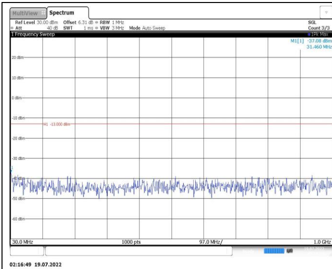
Band25-10MHz-QPSK-26365-1RB#0-Range1:30~1000MHz
