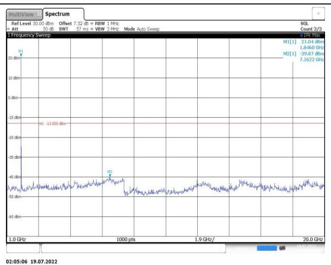
Band25-5MHz-QPSK-26365-1RB#0-Range2:1000~20000MHz
