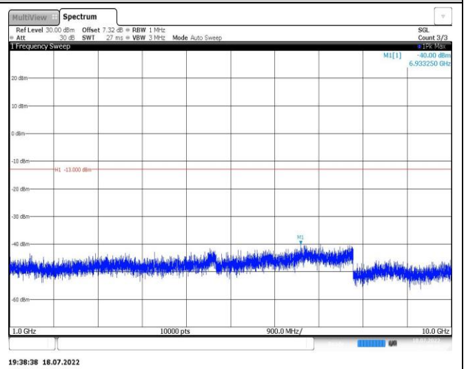
Band12-3MHz-QPSK-23165-1RB#0-Range2:1000~10000MHz
