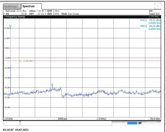
Band25-10MHz-QPSK-26365-1RB#0-Range2:1000~20000MHz
