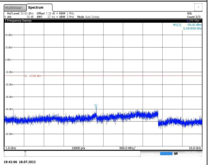
Band12-5MHz-QPSK-23155-1RB#0-Range2:1000~10000MHz
