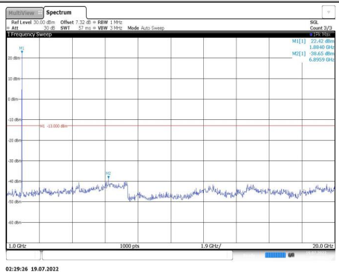
Band25-15MHz-QPSK-26615-1RB#0-Range2:1000~20000MHz
