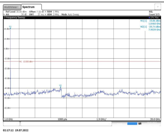
Band25-10MHz-16QAM-26365-1RB#0-Range2:1000~20000MHz
