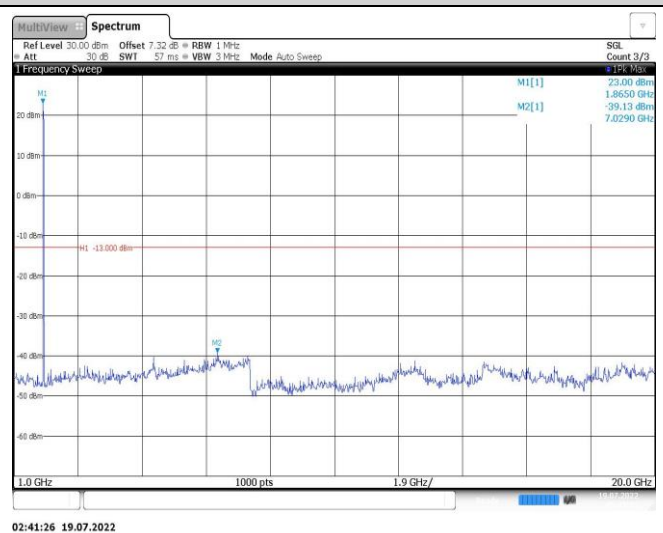
Band25-20MHz-QPSK-26590-1RB#0-Range2:1000~20000MHz
