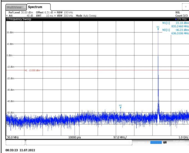
Band26-3MHz-QPSK-27025-1RB#0-Range1:30~1000MHz
