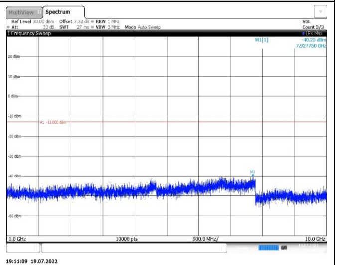
Band26-5MHz-QPSK-26765-1RB#0-Range2:1000~10000MHz
