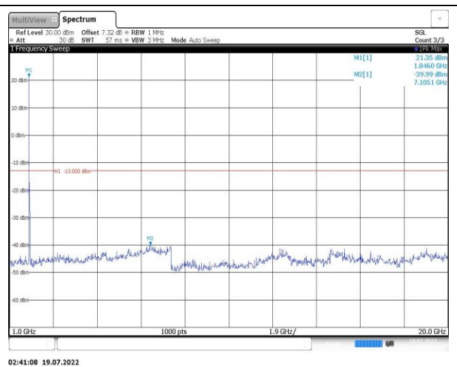
Band25-20MHz-16QAM-26365-1RB#0-Range2:1000~20000MHz
