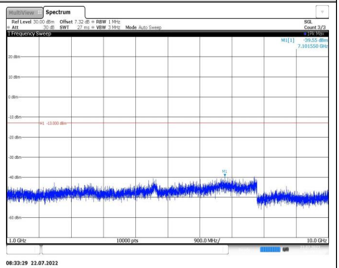
Band26-3MHz-QPSK-27025-1RB#0-Range2:1000~10000MHz
