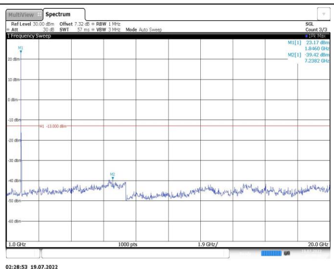
Band25-15MHz-QPSK-26365-1RB#0-Range2:1000~20000MHz
