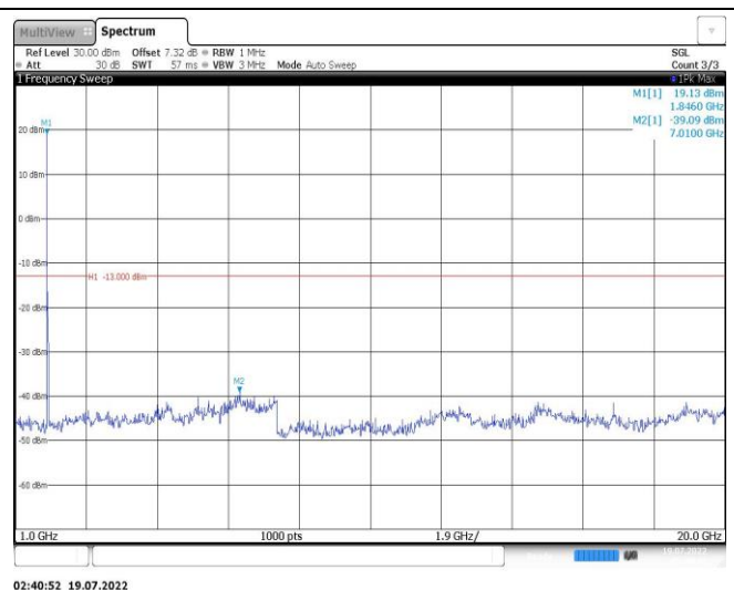
Band25-20MHz-QPSK-26365-1RB#0-Range2:1000~20000MHz
