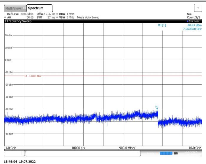
Band26-1.4MHz-QPSK-26797-1RB#0-Range2:1000~10000MHz
