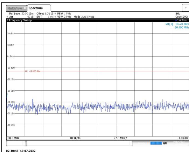
Band25-20MHz-QPSK-26365-1RB#0-Range1:30~1000MHz
