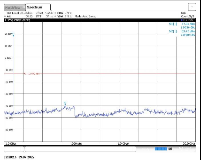
Band25-20MHz-QPSK-26140-1RB#0-Range2:1000~20000MHz
