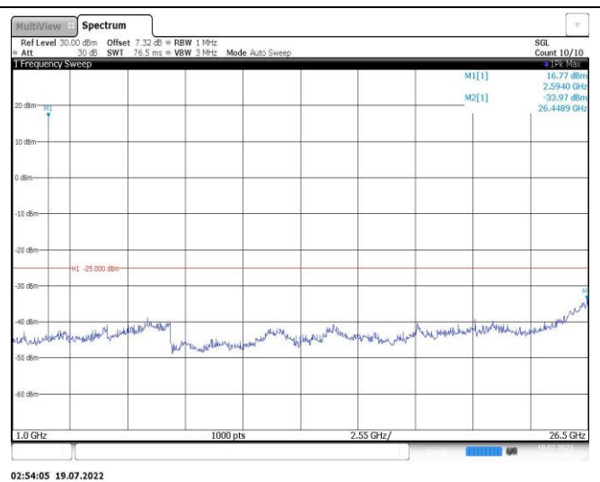
Band38-5MHz-QPSK-38225-1RB#0-Range2:1000~26500MHz
