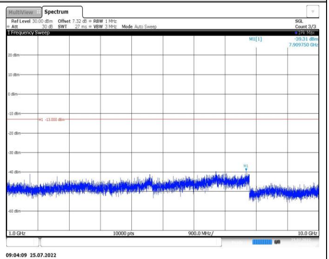
Band26-10MHz-QPSK-26990-1RB#0-Range2:1000~10000MHz
