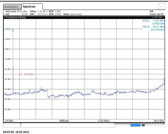
Band41-10MHz-QPSK-40620-1RB#0-Range2:1000~26500MHz
