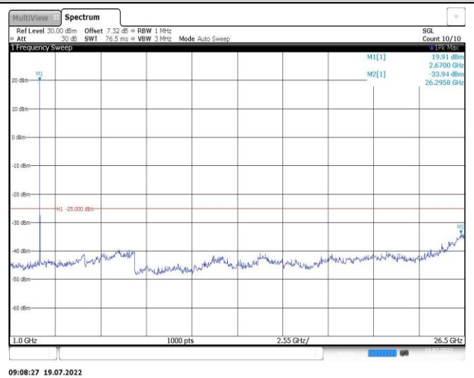
Band41-15MHz-QPSK-39725-1RB#0-Range2:1000~26500MHz
