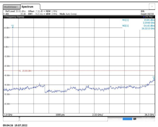
Band41-5MHz-QPSK-41565-1RB#0-Range2:1000~26500MHz
