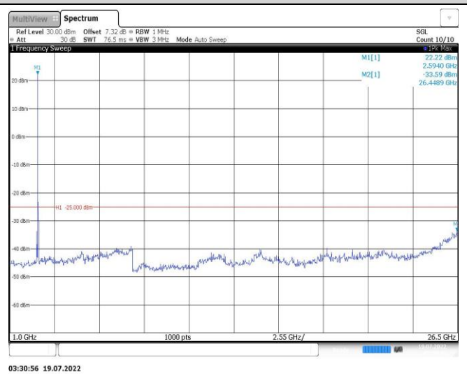
Band41-5MHz-QPSK-39675-1RB#0-Range2:1000~26500MHz
