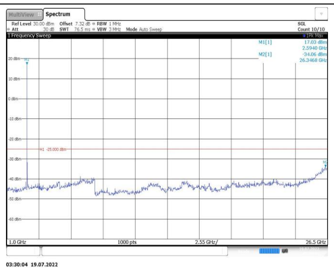
Band38-20MHz-QPSK-38150-1RB#0-Range2:1000~26500MHz
