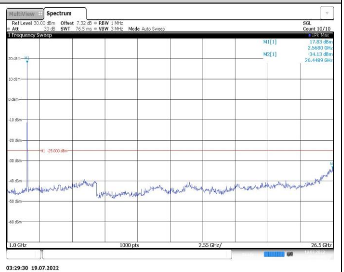
Band38-20MHz-QPSK-38000-1RB#0-Range2:1000~26500MHz
