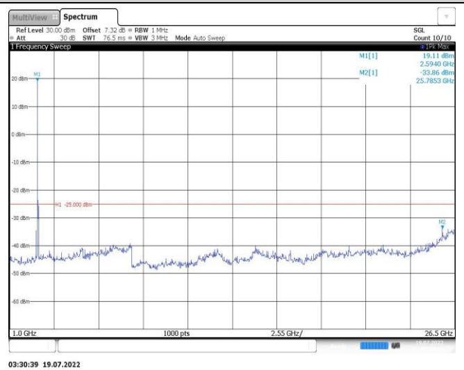
Band38-20MHz-16QAM-37850-1RB#0-Range2:1000~26500MHz
