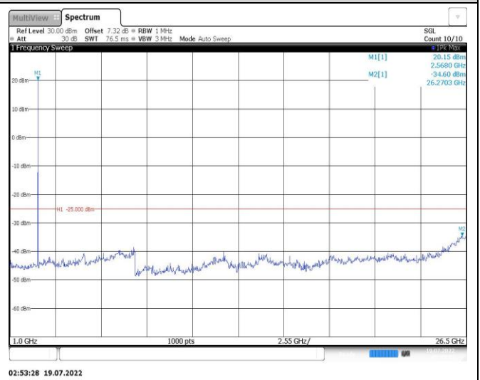
Band38-5MHz-QPSK-38000-1RB#0-Range2:1000~26500MHz
