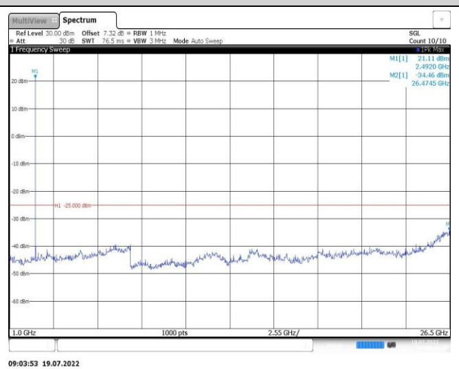
Band41-5MHz-QPSK-40620-1RB#0-Range2:1000~26500MHz
