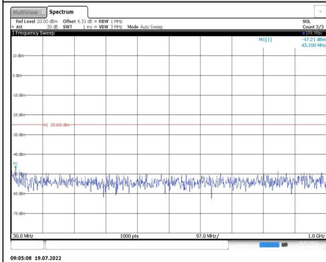
Band41-10MHz-QPSK-39700-1RB#0-Range1:30~1000MHz
