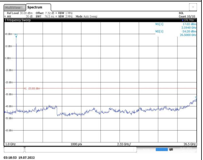
Band38-20MHz-QPSK-37850-1RB#0-Range2:1000~26500MHz
