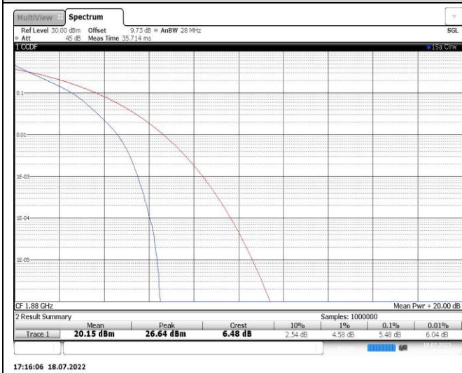
Band2-5MHz-QPSK-18900-25RB#0
