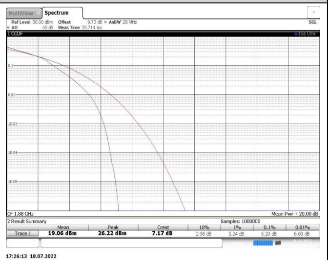
Band2-20MHz-16QAM-18900-100RB#0
