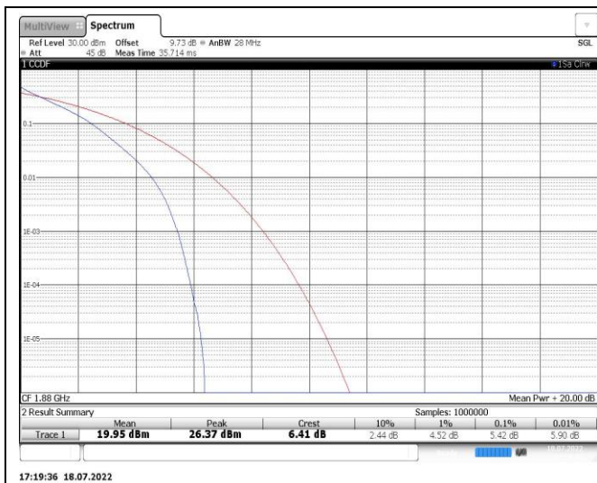
Band2-10MHz-QPSK-18900-50RB#0
