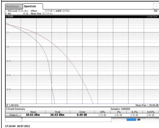
Band2-20MHz-QPSK-18900-100RB#0
