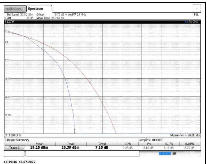
Band2-10MHz-16QAM-18900-50RB#0
