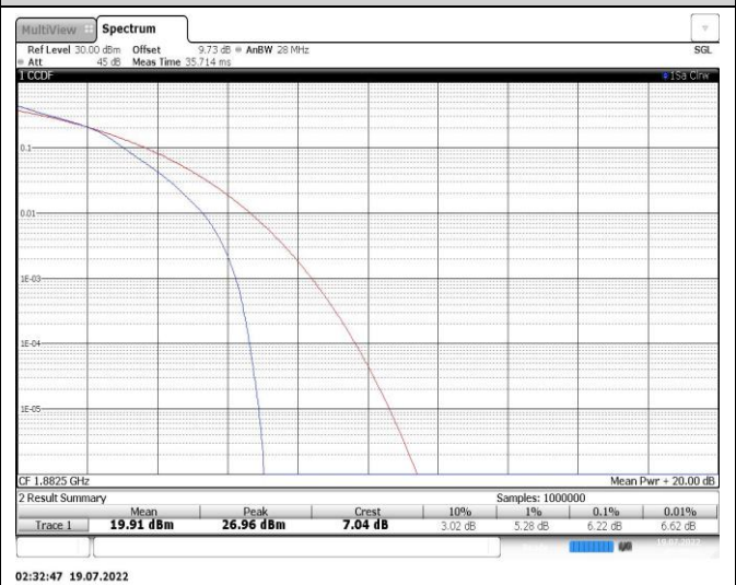
Band25-20MHz-16QAM-26365-100RB#0
