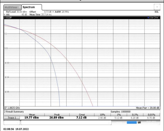
Band25-10MHz-16QAM-26365-50RB#0
