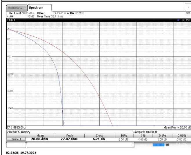
Band25-20MHz-QPSK-26365-100RB#0
