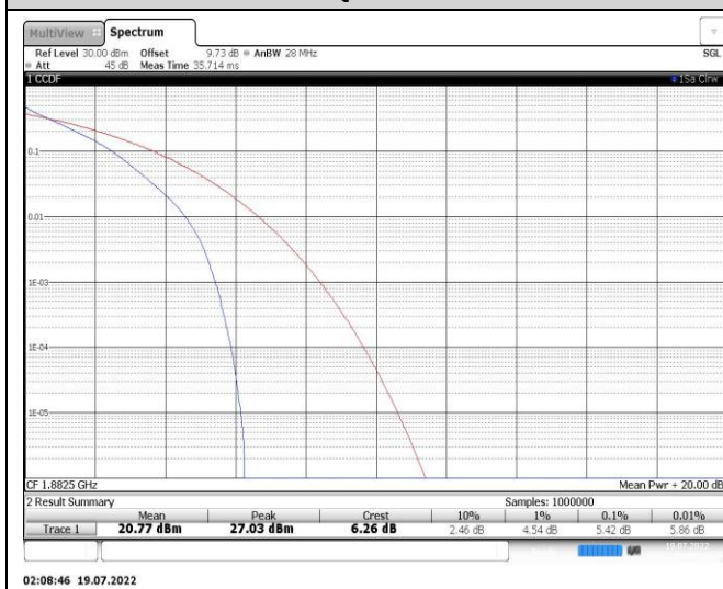
Band25-10MHz-QPSK-26365-50RB#0
