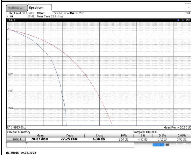
Band25-5MHz-QPSK-26365-25RB#0
