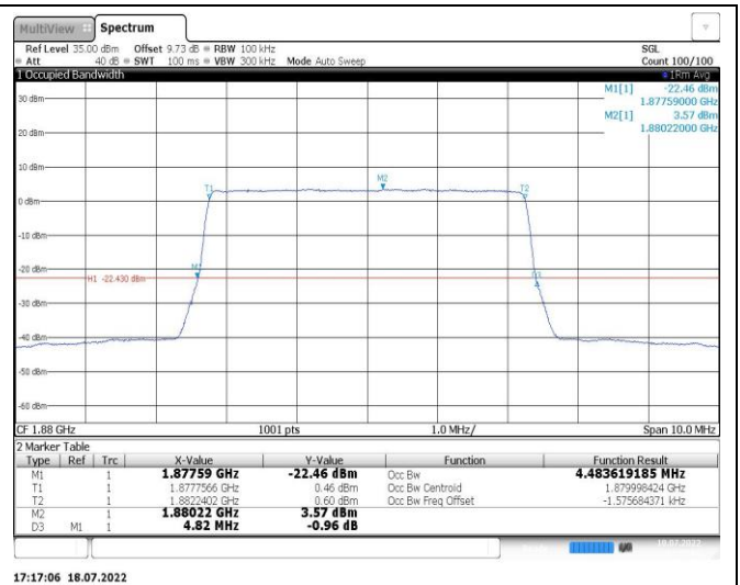
Band2-10MHz-16QAM-18900-50RB#0
