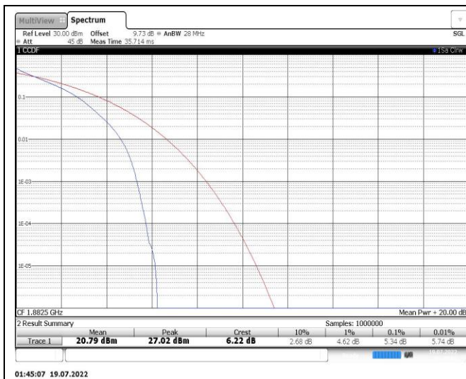
Band25-3MHz-QPSK-26365-15RB#0
