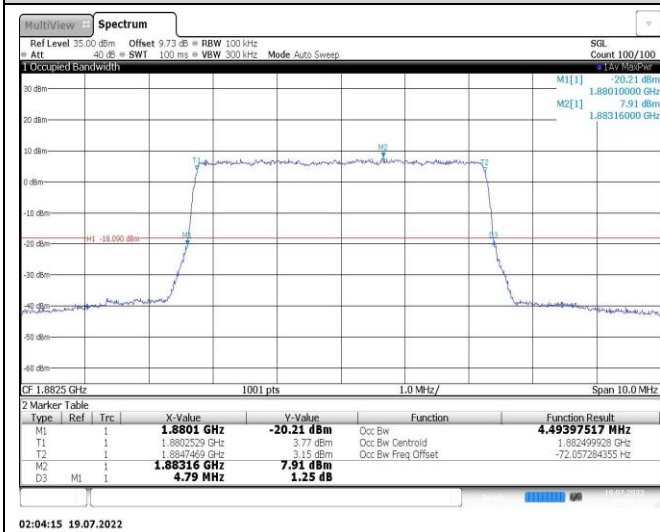
Band25-10MHz-QPSK-26365-50RB#0
