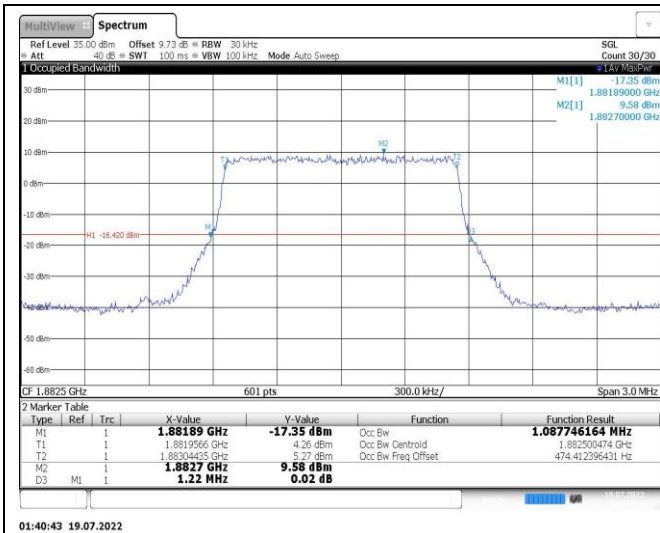
Band25-3MHz-QPSK-26365-15RB#0
