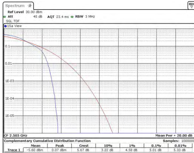
Band7-10MHz-QPSK-20800-50RB#0
