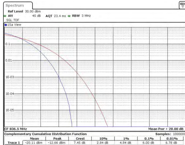
Band5-3MHz-QPSK-20635-1RB#0
