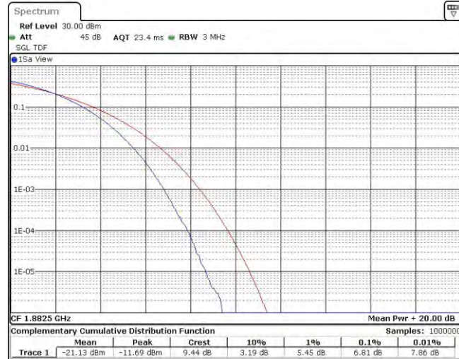
Band25-3MHz-QPSK-26365-15RB#0
