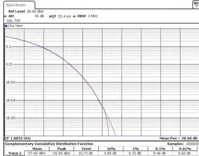
Band25-20MHz-16QAM-26365-100RB#0
