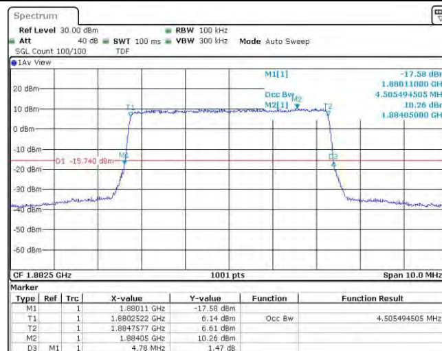
Band25-5MHz-QPSK-26365-25RB#0
