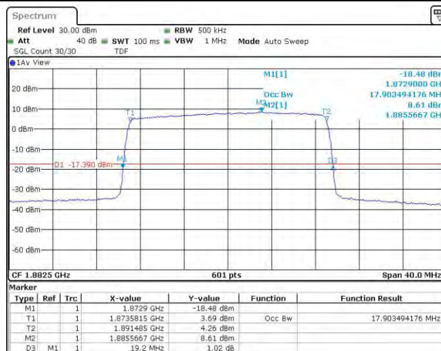
Band25-20MHz-16QAM-26365-100RB#0
