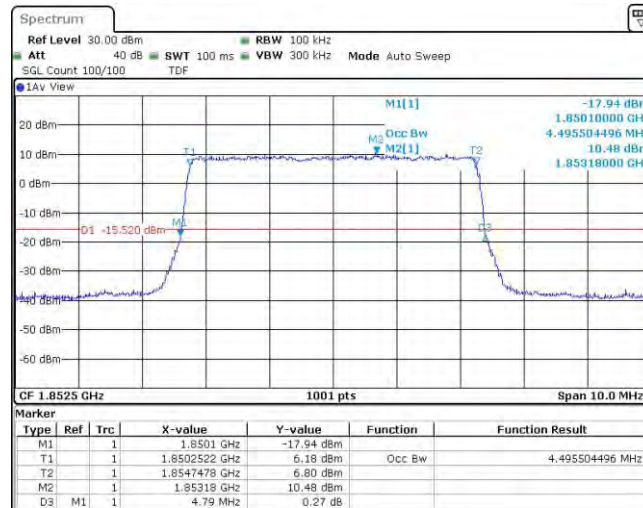
Band25-5MHz-QPSK-26365-25RB#0
