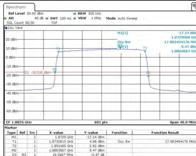
Band25-20MHz-QPSK-26365-100RB#0
