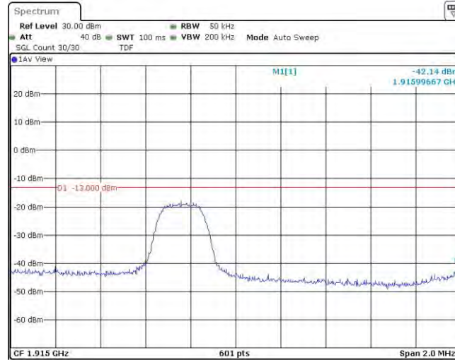
Band25-3MHz-QPSK-26675-1RB#14
