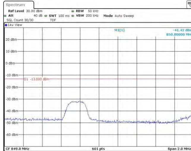
Band5-3MHz-QPSK-20635-1RB#14
