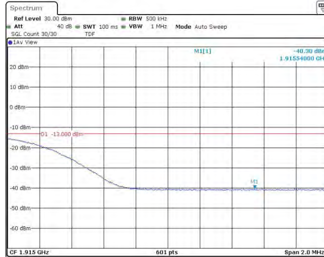
Band25-20MHz-16QAM-26590-1RB#99
