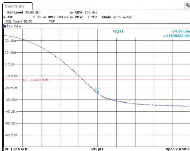
Band25-20MHz-QPSK-26590-100RB#0
