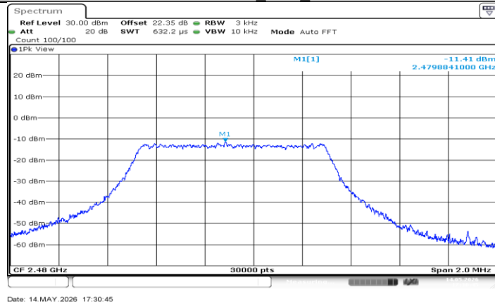
CSS 812kHz_Ant1_2480
