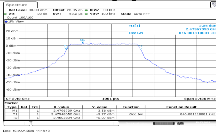
CSS 812kHz_Ant1_2480
