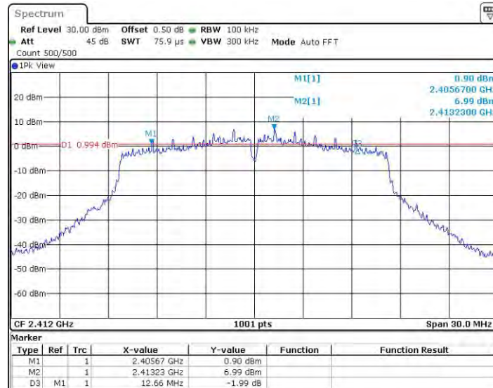
11G_Ant2_2412
