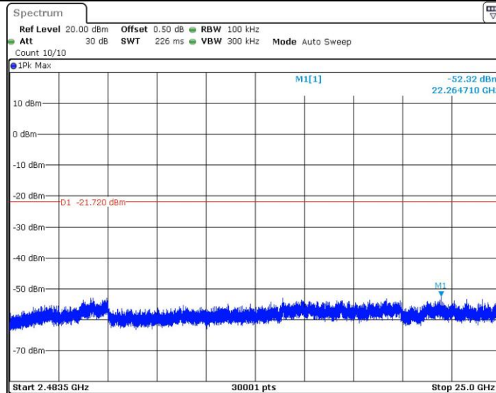
BLE_2M_2402_2483.5~25000
