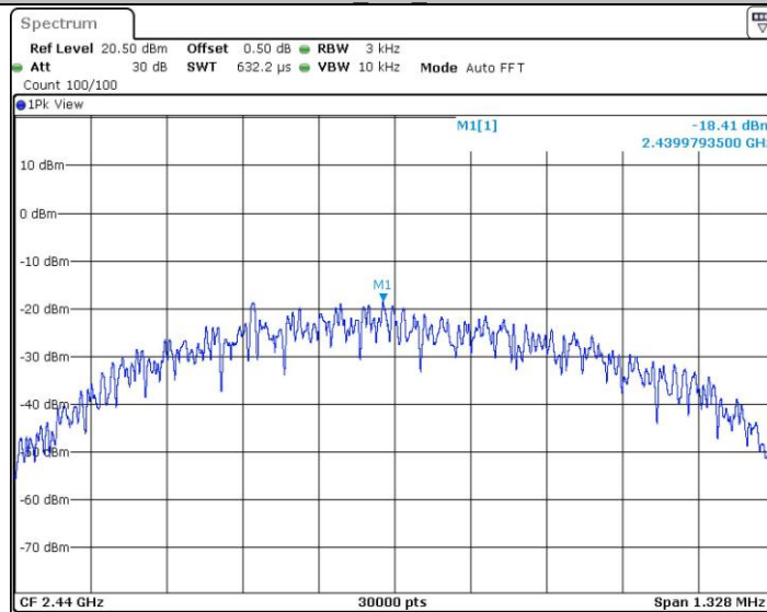
BLE 1M 2440
