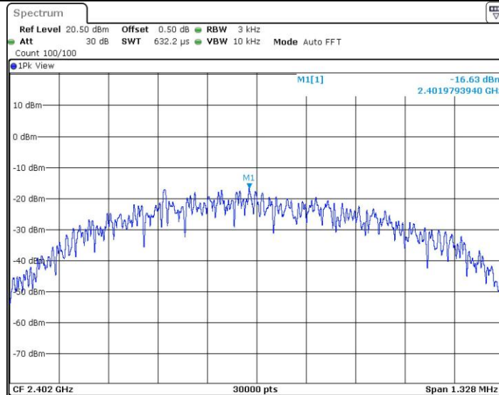
BLE 1M 2402
