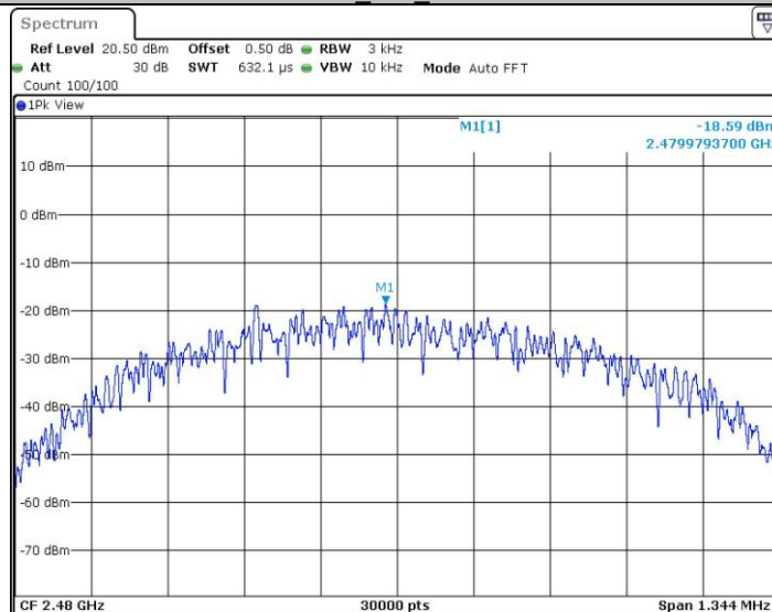
BLE 1M 2480
