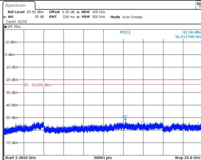
BLE 2M 2480 2483.5~25000
