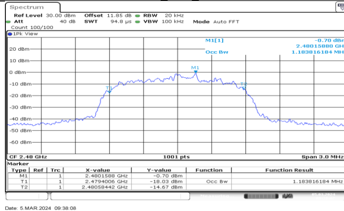
3DH5 Ant1 2480
