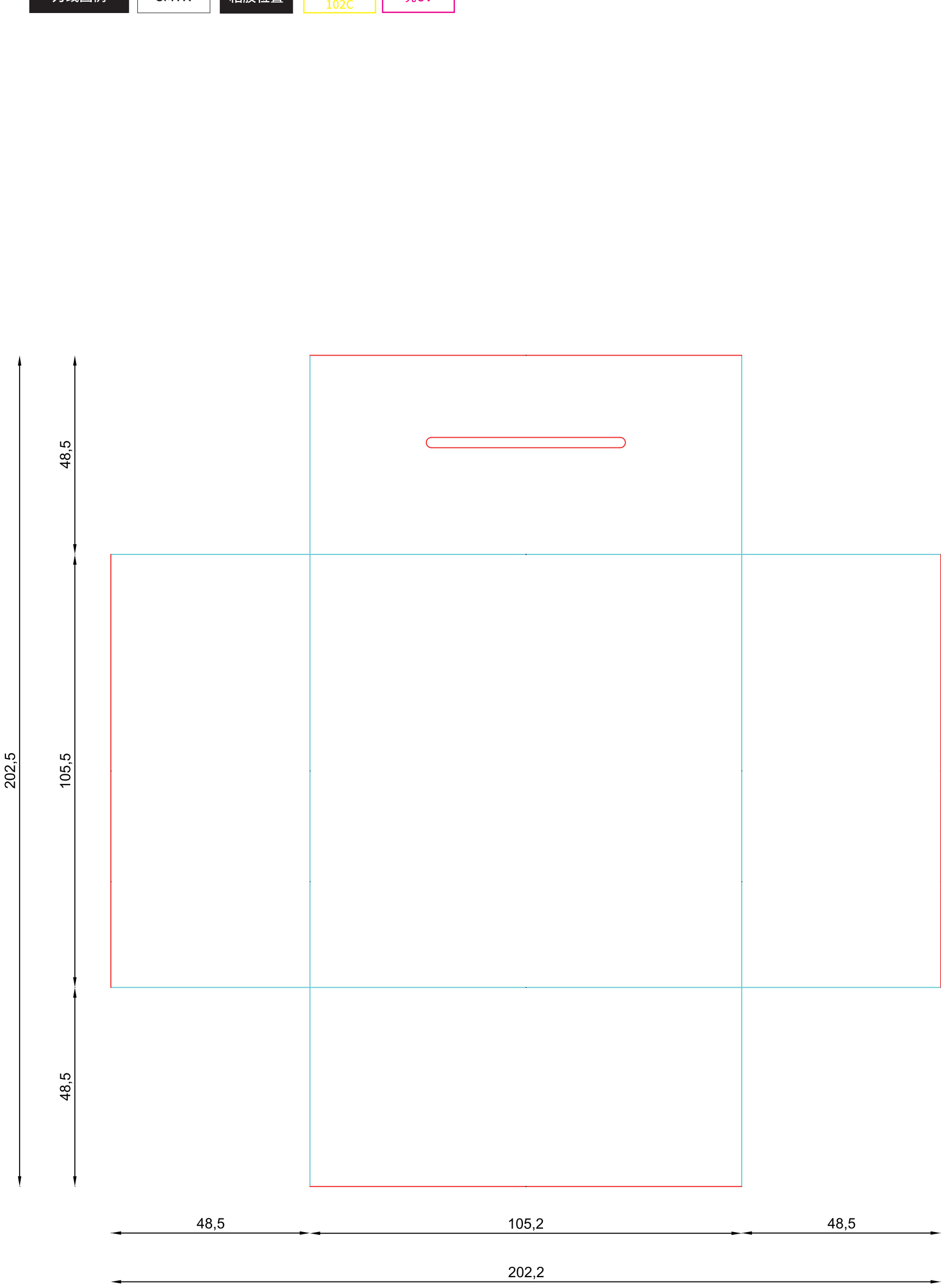
天盒：800G 厚单面白灰板，V90 度
