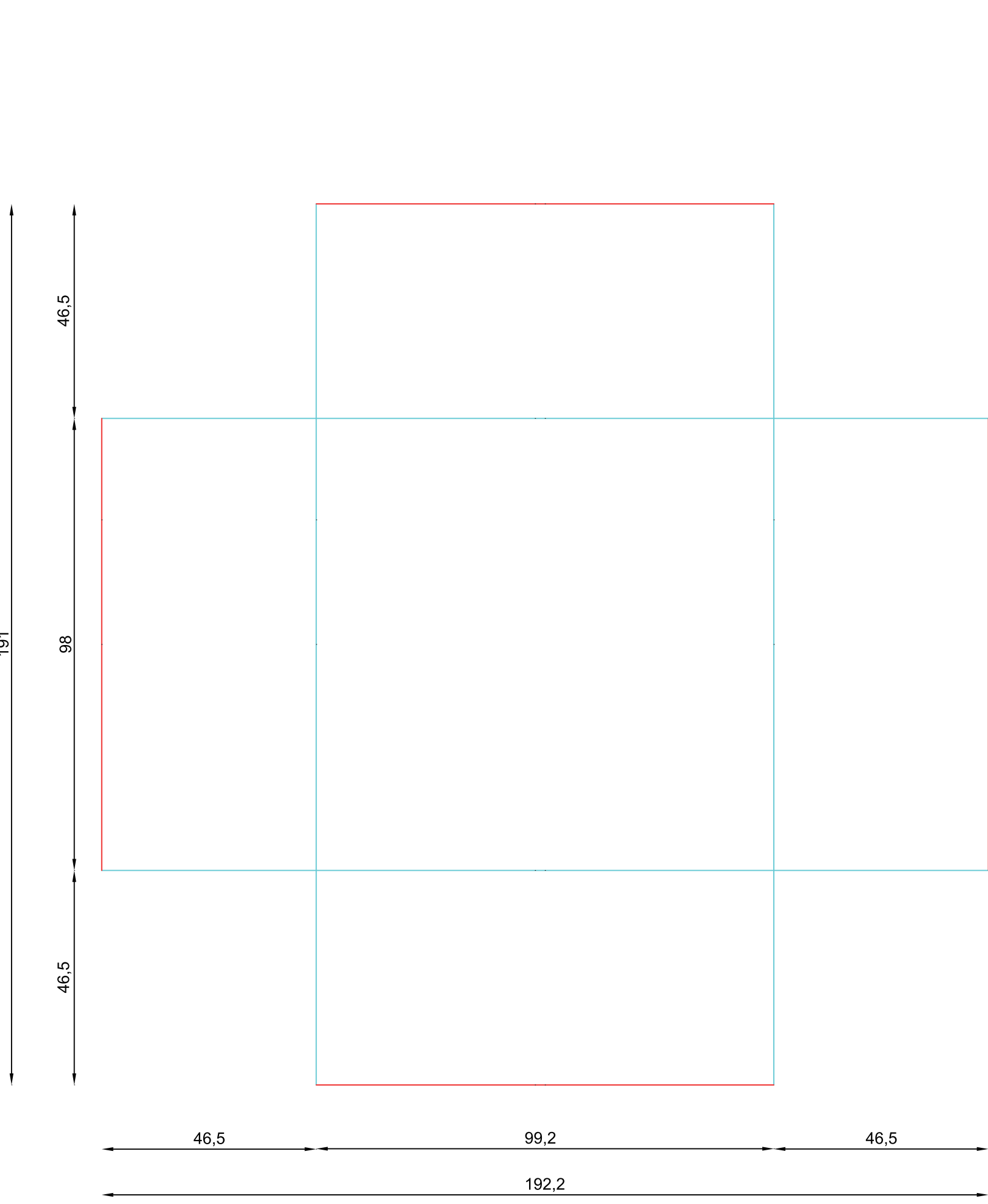
地盒：800G 厚单面白灰板，V90 度
