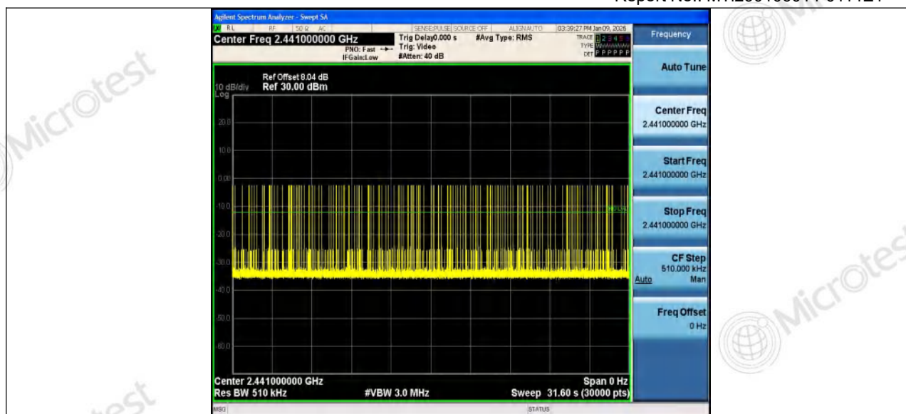
DH3_Ant2_Hop
