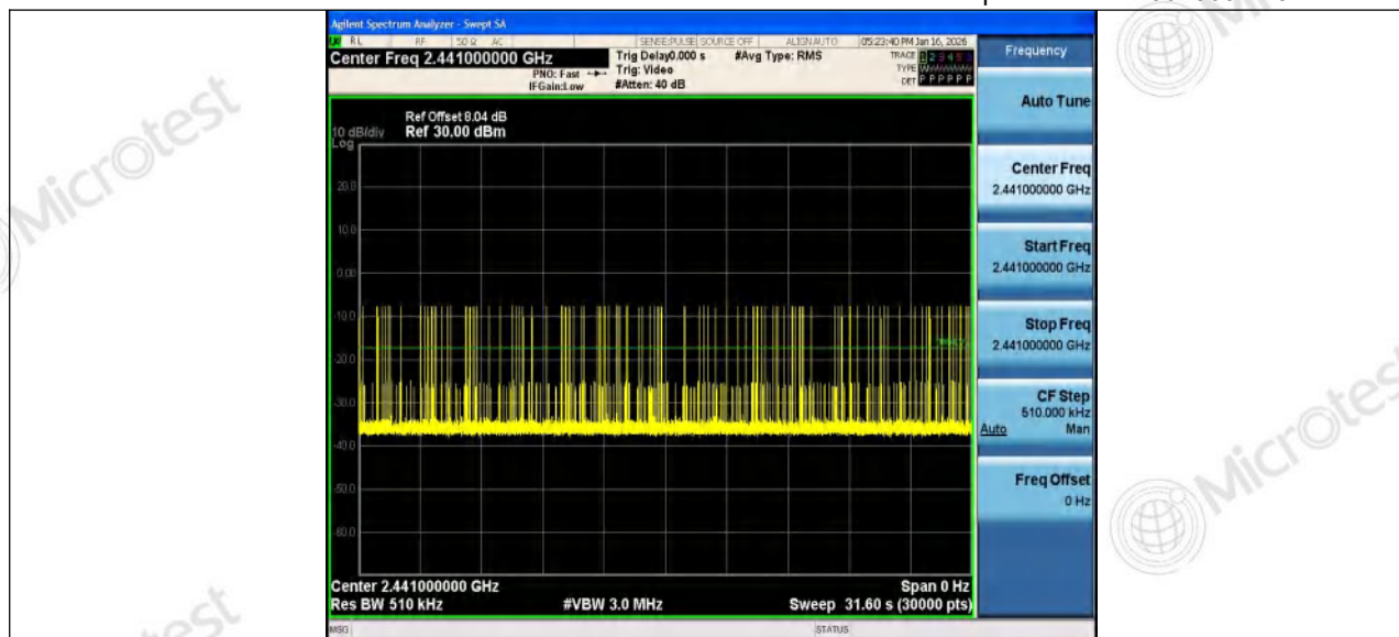
3DH1_Ant1_Hop
