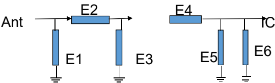
匹配电路图
