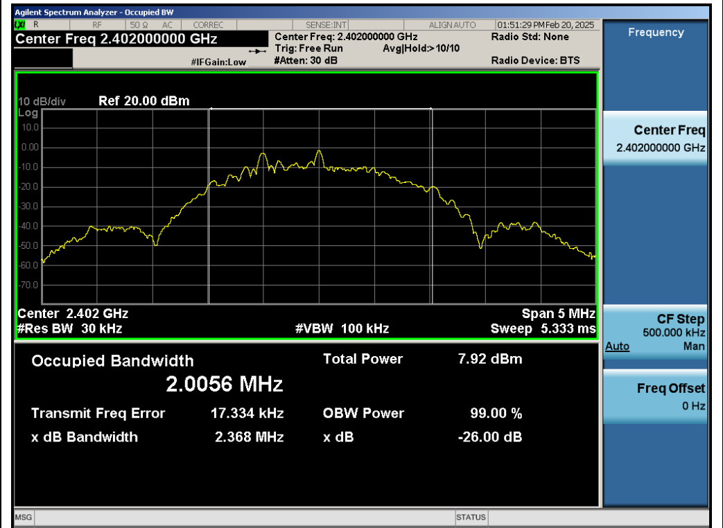
Test_Graph_LE2M_ANT1_2402_2Mbps_OBW
