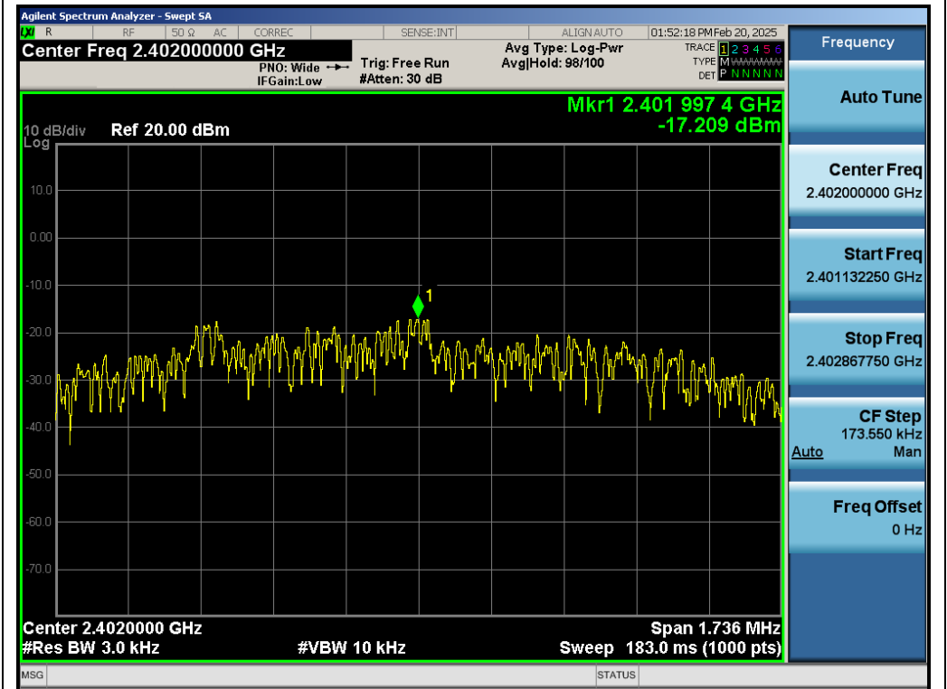
Test_Graph_LE2M_ANT1_2402_2Mbps_PSD
