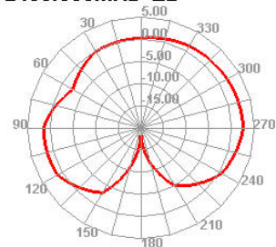
2400.000MHz E2
