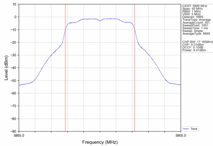
802.11a_HCH_5885MHz_Ant1_NTNV
