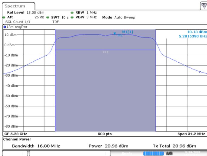
SISO B-802.11a-20MHz-Ch56-5280MHz-6
