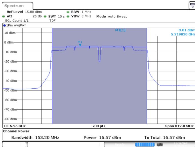
SISO A-802.11ac-160MHz-Ch50-5250MHz-VHT0
