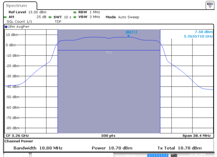
MIMO B-802.11ax-20MHz-Ch52-5260MHz-HE0
