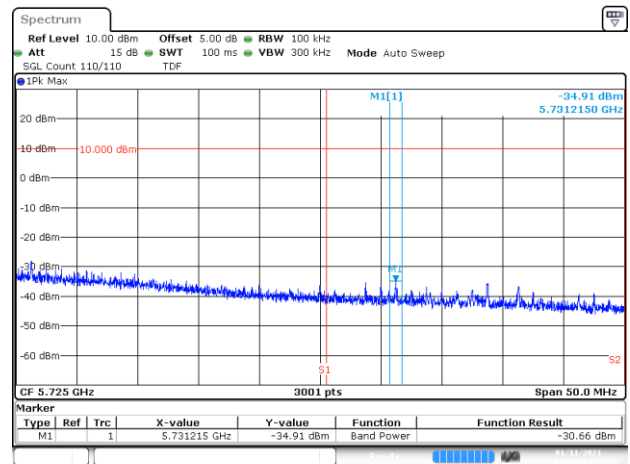
BE-NR-HIGH, MIMO-B, 802.11ax40-HE0, Ch134
