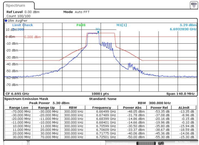
SISO-B, 802.11ax/be20-MCS0, Ch149-8m-53
