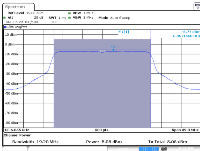
SISO B-802.11ax-20MHz-Ch181-6855MHz-HE0
