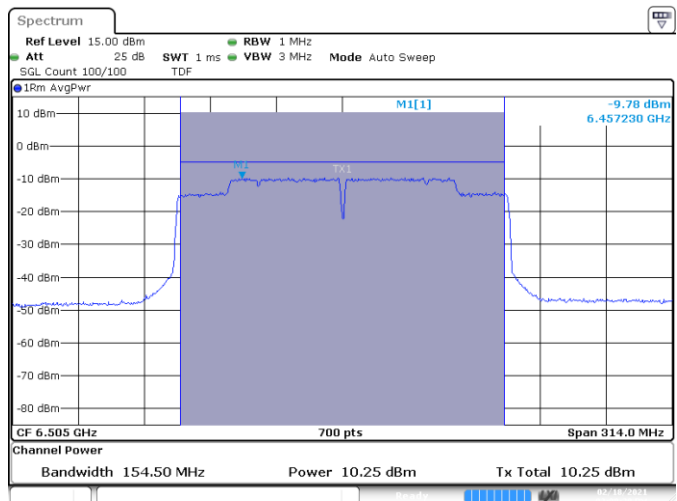
MIMO B-802.11ax-160MHz-Ch111-6505MHz-HE0
