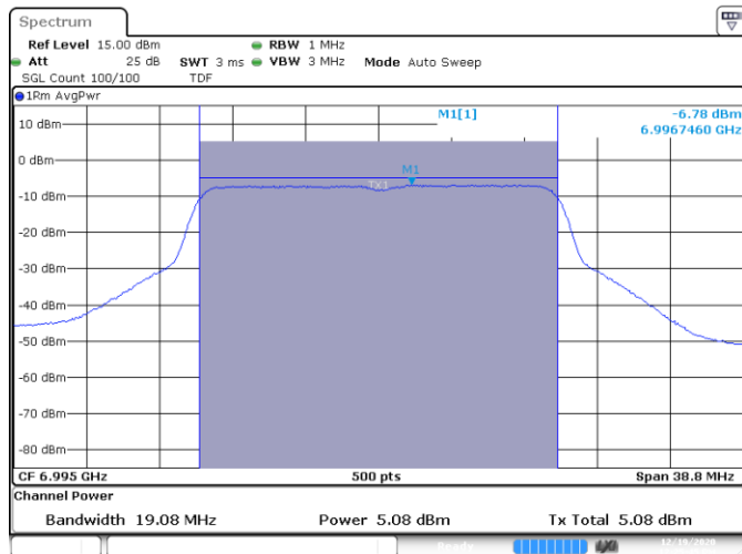
SISO B-802.11ax-20MHz-Ch209-76995MHz-HE0
