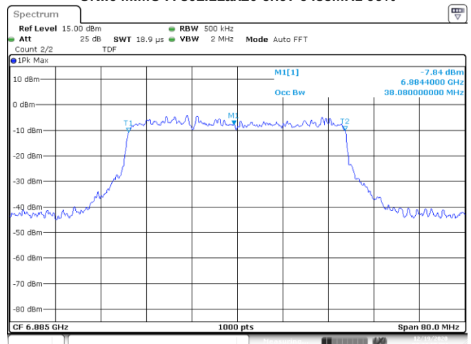
UNII8 MIMO A 802.11ax40 ch187 6885MHz 99%
