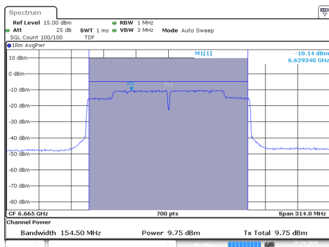
MIMO B-802.11ax-160MHz-Ch143-6665MHz-HE0
