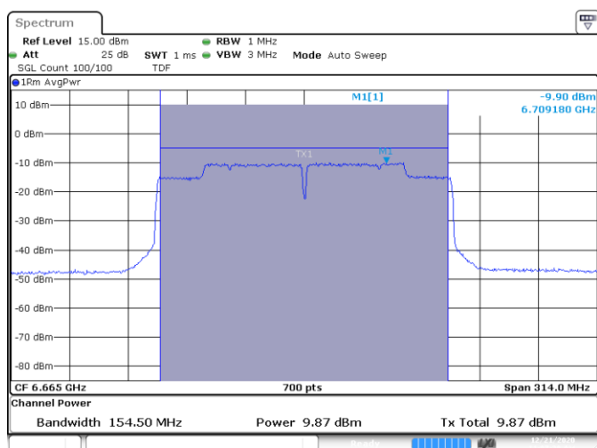
MIMO A-802.11ax-160MHz-Ch143-6665MHz-HE0
