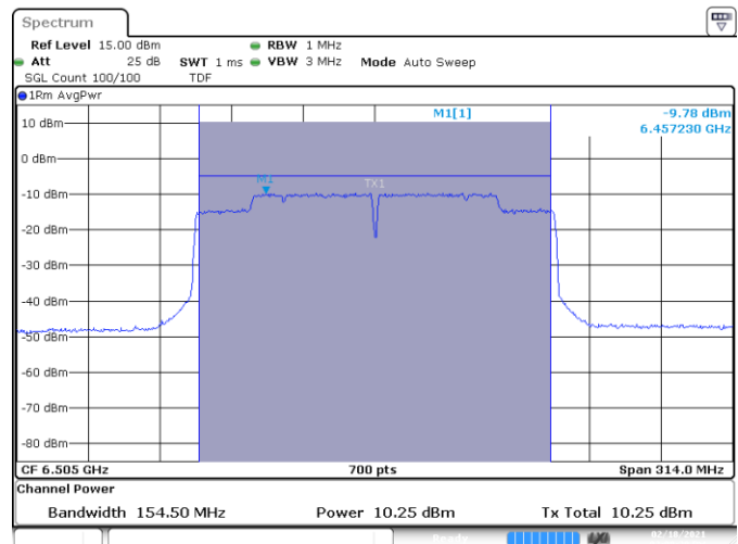
MIMO B-802.11ax-160MHz-Ch111-6505MHz-HE0
