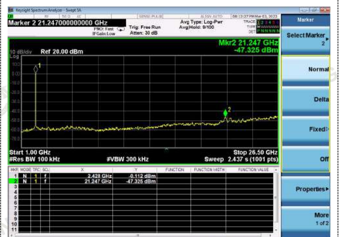
1GHz -26.5GHz
