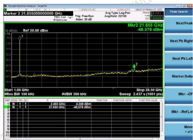
1GHz -26.5GHz
