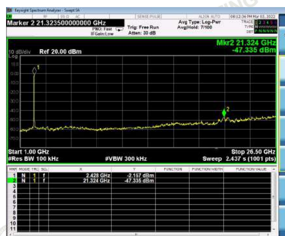
1GHz -26.5GHz
