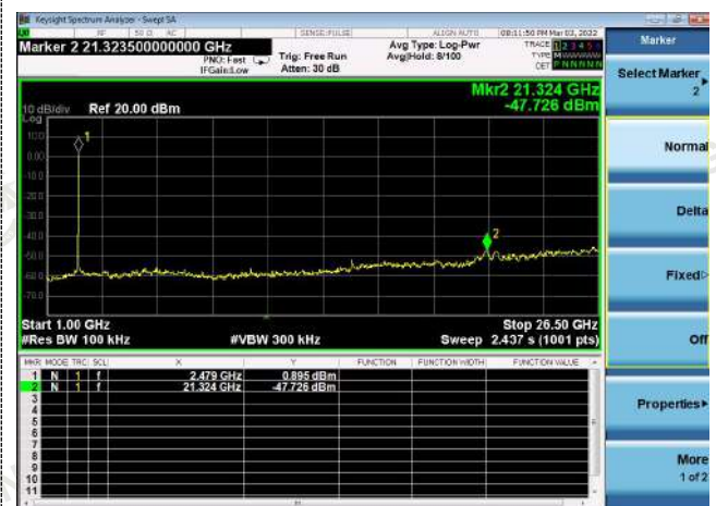
1GHz -26.5GHz
