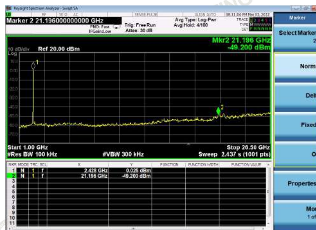
1GHz -26.5GHz
