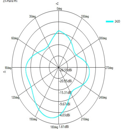
ZX-Plane Phi
