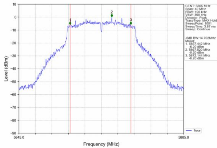
802.11a_LCH_5865MHz_Ant1_NTNV
