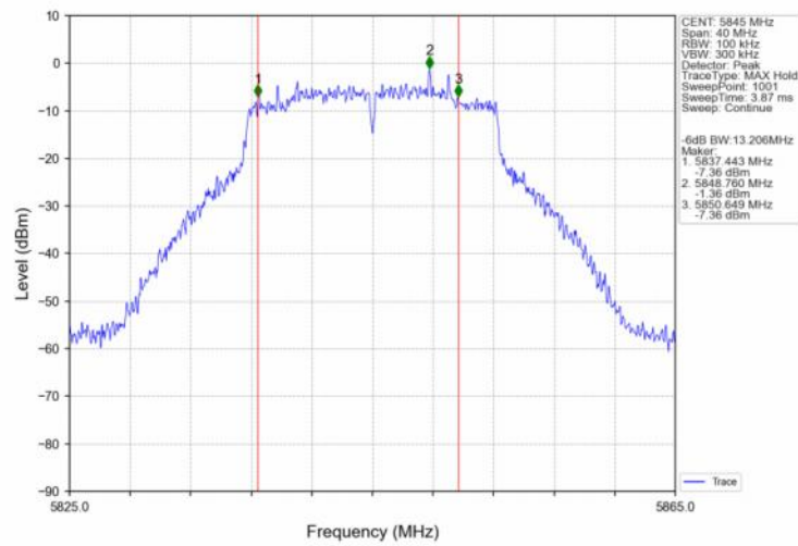
802.11a_HCH_5845MHz_Ant1_NTNV
