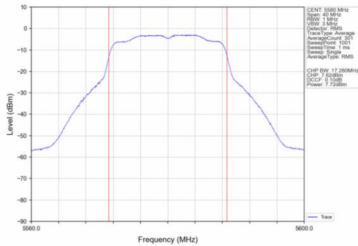
802.11a_MCH_5580MHz_Ant2_NTNV
