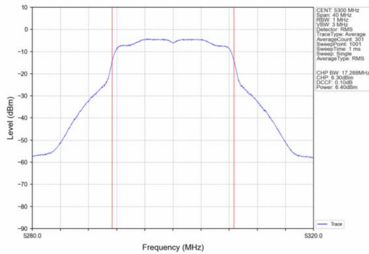
802.11a_MCH_5300MHz_Ant2_NTNV
