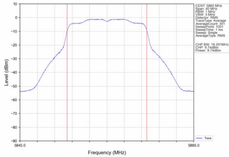
802.11n(HT20)_LCH_5865MHz_Ant2_NTNV
