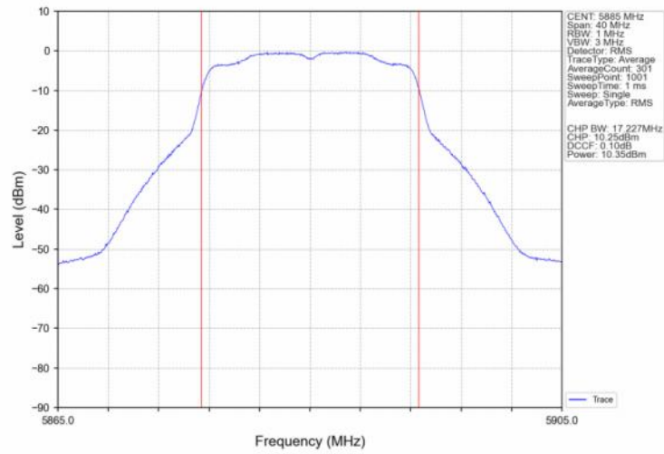
802.11a_HCH_5885MHz_Ant2_NTNV
