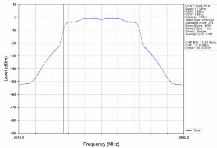
802.11n(HT20)_LCH_5865MHz_Ant2_NTNV
