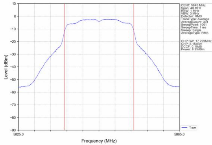
802.11a_HCH_5845MHz_Ant2_NTNV
