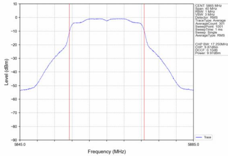
802.11a_LCH_5865MHz_Ant2_NTNV
