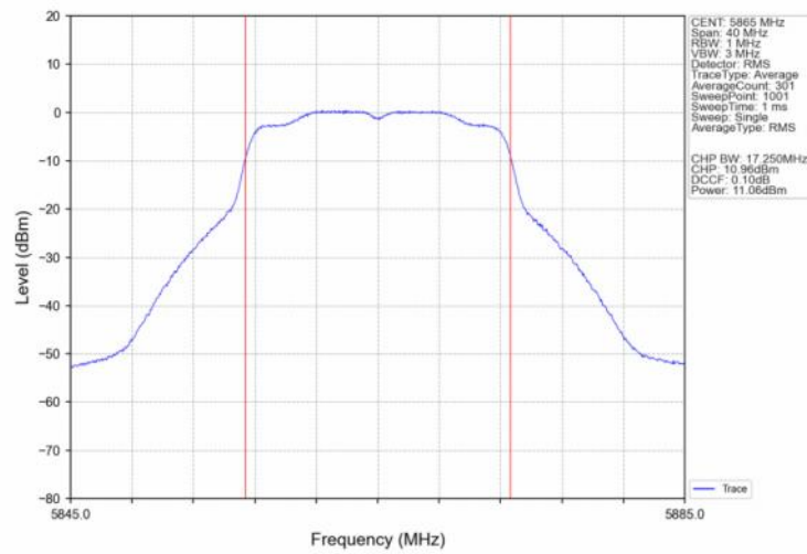
802.11a_LCH_5865MHz_Ant2_NTNV
