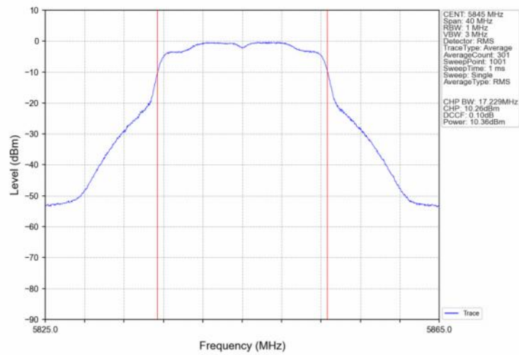
802.11a_HCH_5845MHz_Ant2_NTNV
