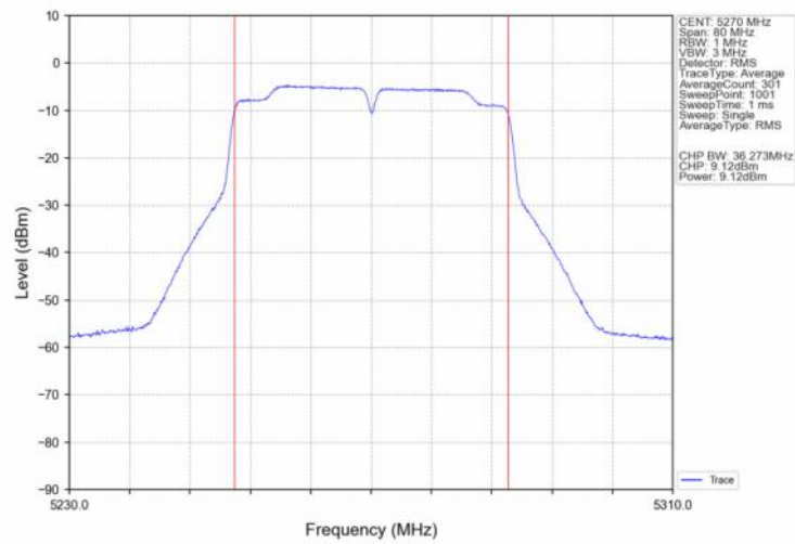
802.11n(HT40)_LCH_5270MHz_Ant2_NTNV
