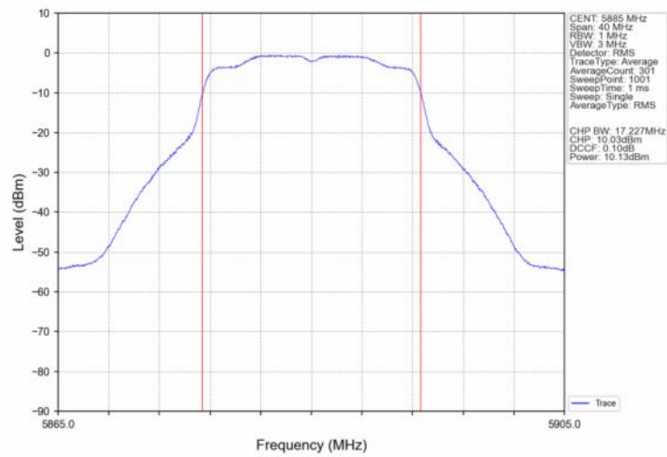
802.11a_HCH_5885MHz_Ant2_NTNV
