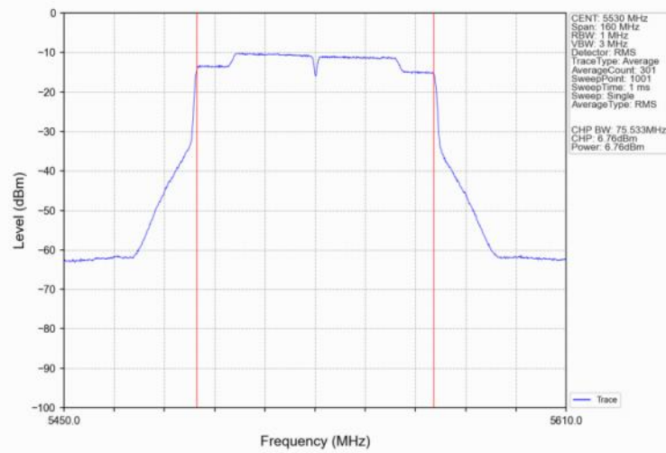
802.11ac(VHT80)_LCH_5530MHz_Ant2_NTNV
