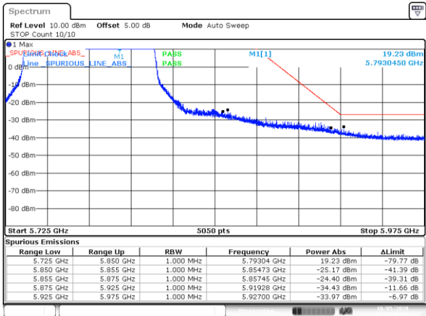
BE-NR-HIGH, MIMO-A, 802.11ac80-HE0, Ch155
