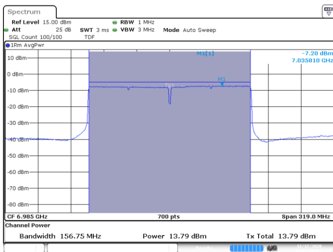
SISO A-802.11ax-160MHz-Ch207-6985MHz-HE0
