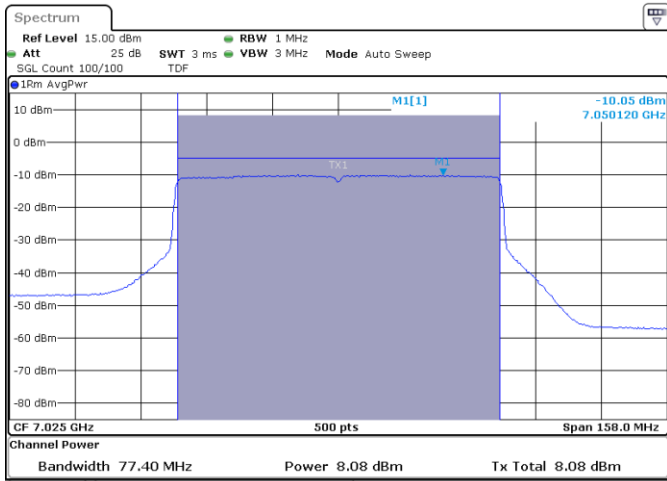
MIMO A-802.11ax-80MHz-Ch215-7025MHz-HE0
