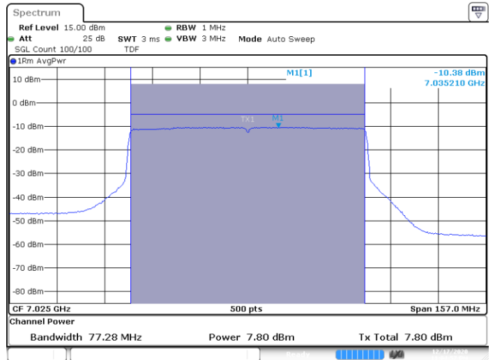
MIMO B-802.11ax-80MHz-Ch215-7025MHz-HE0
