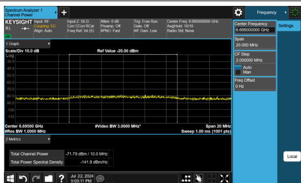
802.11ax-HE20 / CH149
